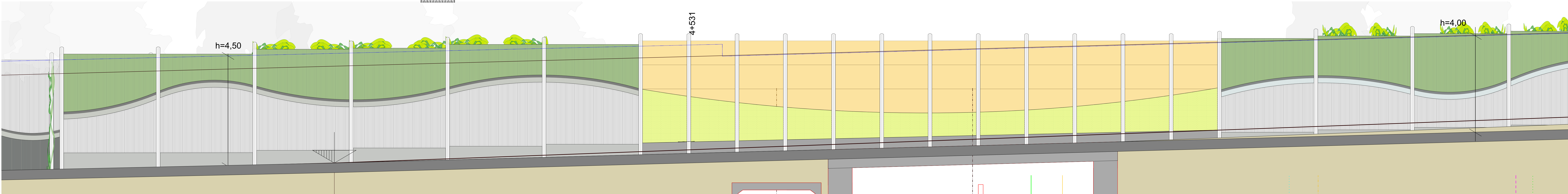
Ansicht LSW im Bereich Unterführung - LSW 1 M 1 / 50
