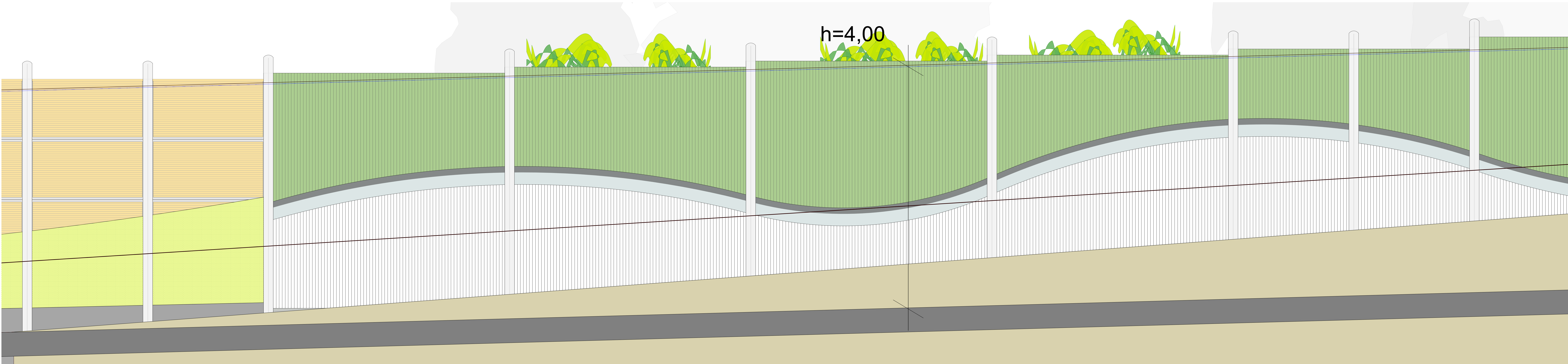
Ansicht LSW - LSW 1 M 1 / 20
