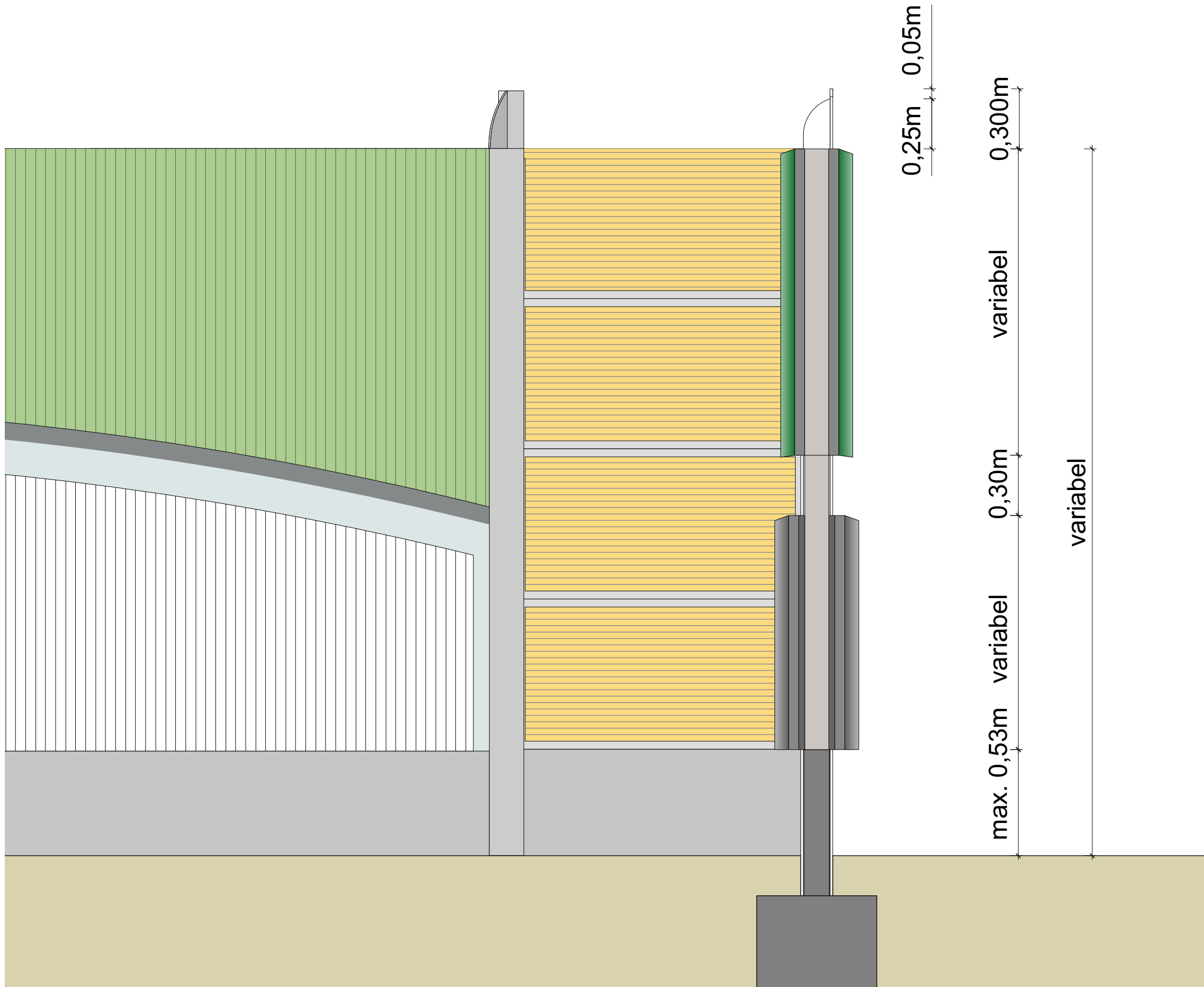
Ansicht / Schnitt LSW mit Fenster LSW 1 M 1 / 20
