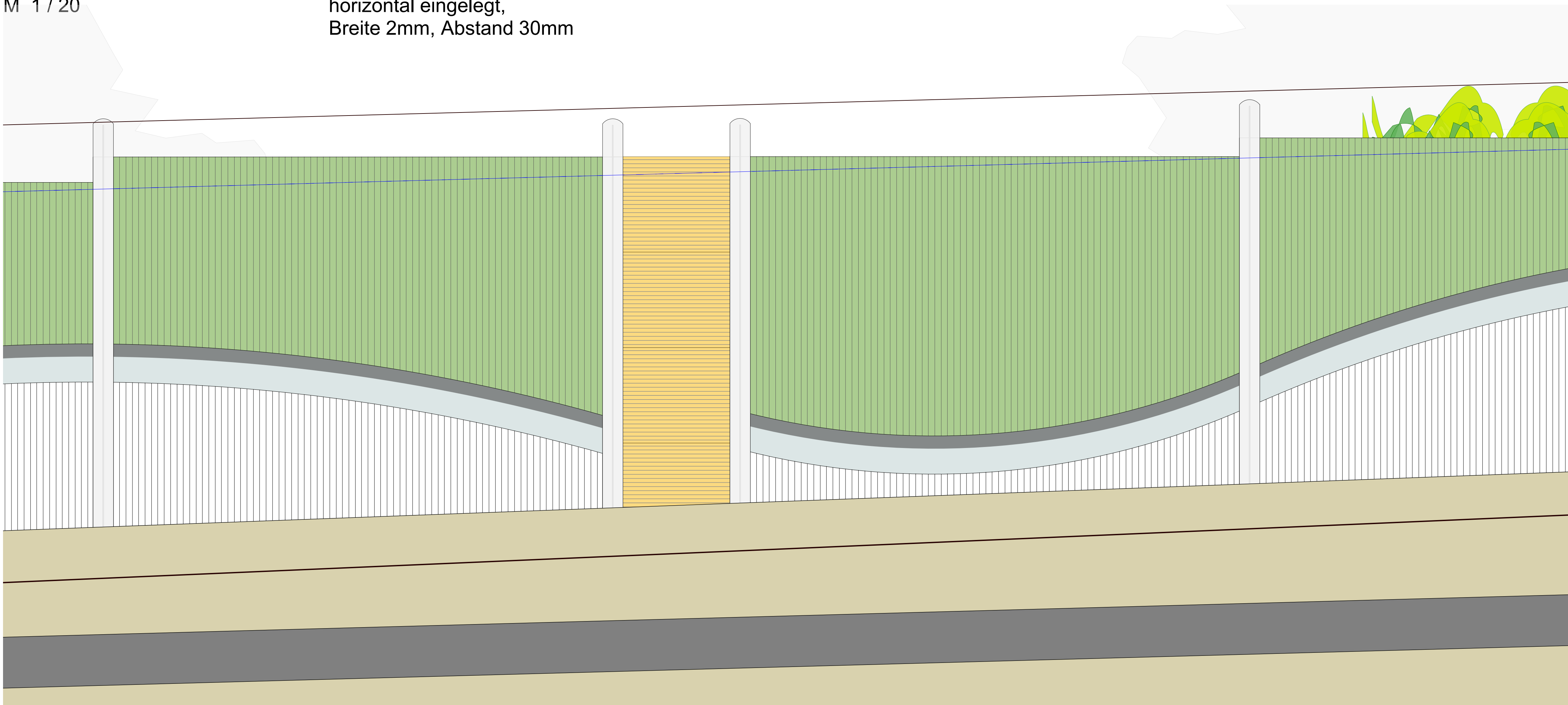
Ausschnitt Abwicklung LSW mit Fenster LSW 1 M 1 / 20
