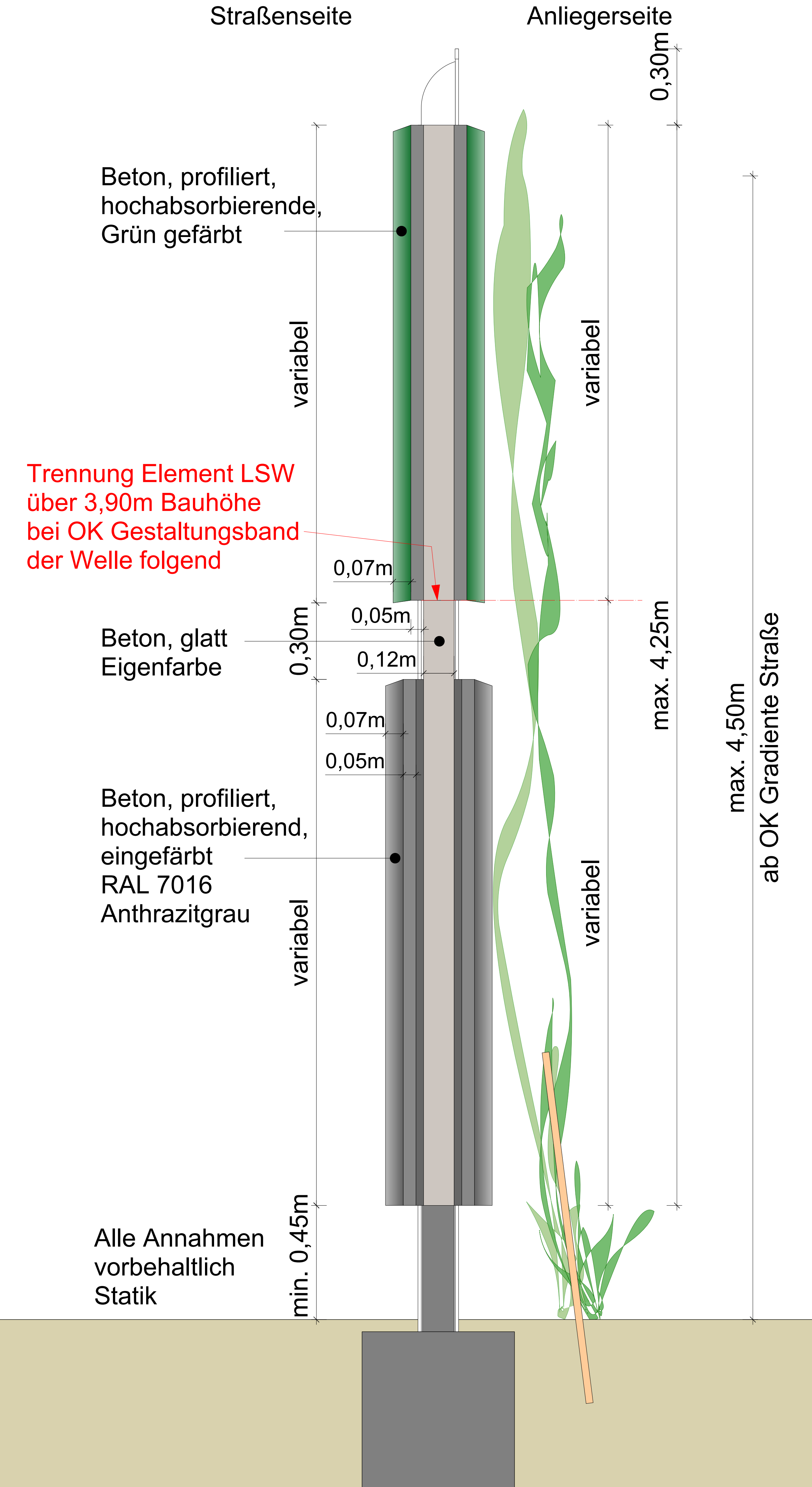
Schnitt LSW 1 M 1 / 10
