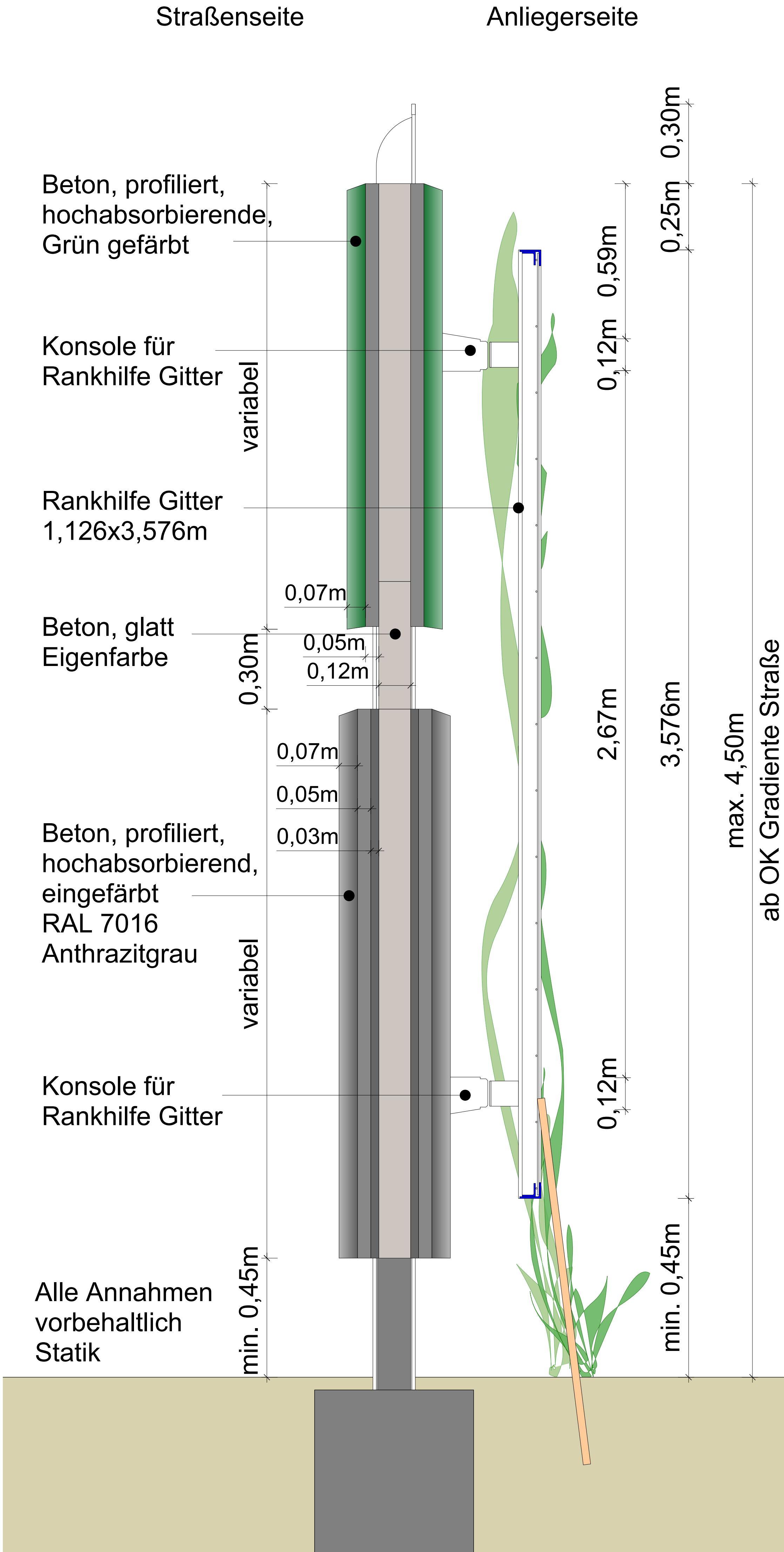
Schnitt mit Rankhilfe LSW 1 M 1 / 10
