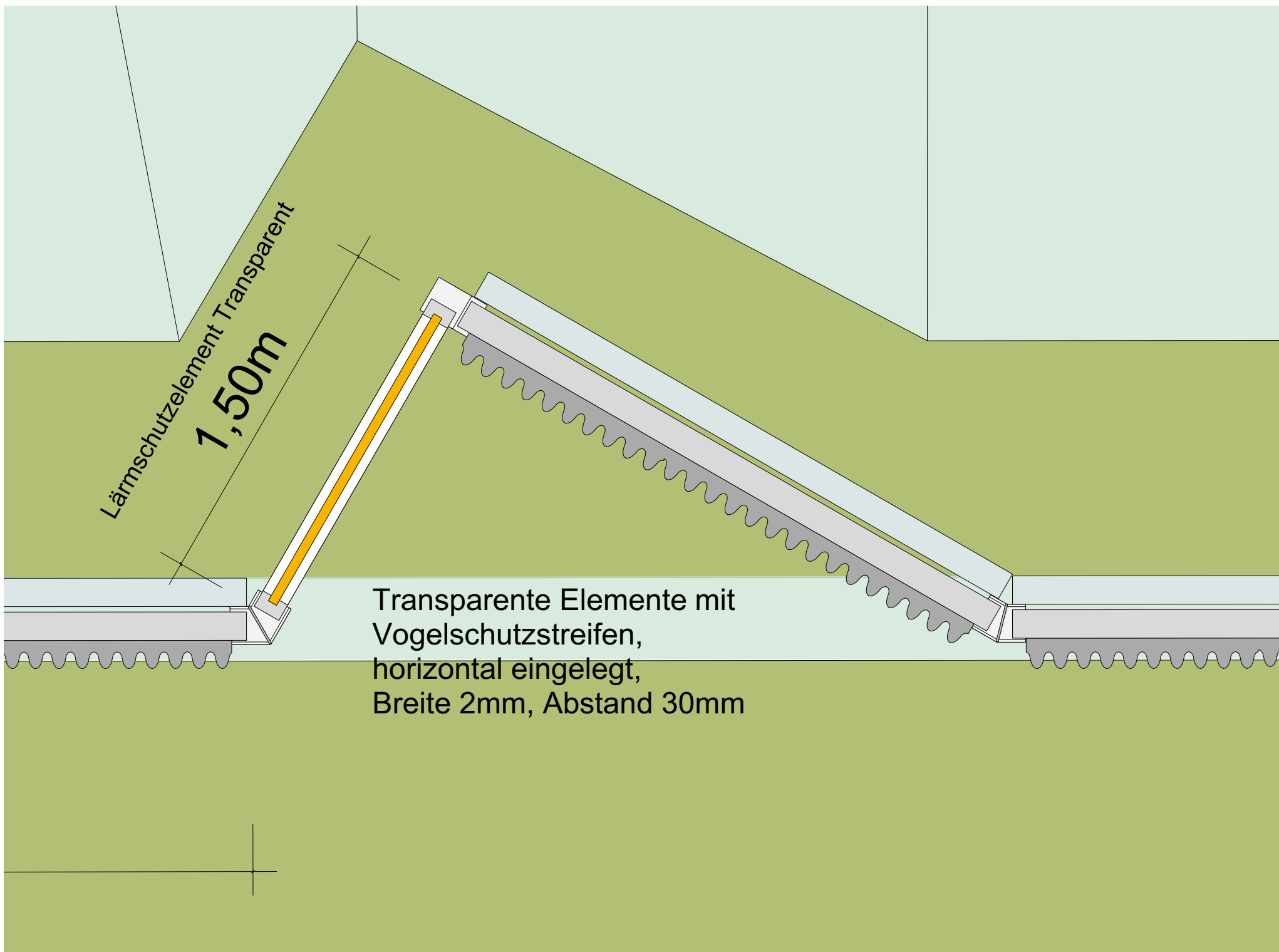
Schema LSW mit Fenster - LSW 4 M 1 / 20
