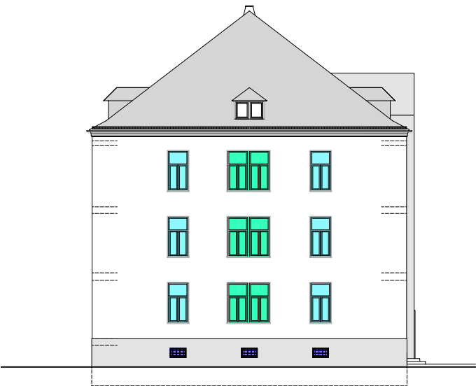
ANSICHT SÜD-OSTEN (Seitenansicht)
