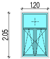
Fenster typ 1 30 Stk
