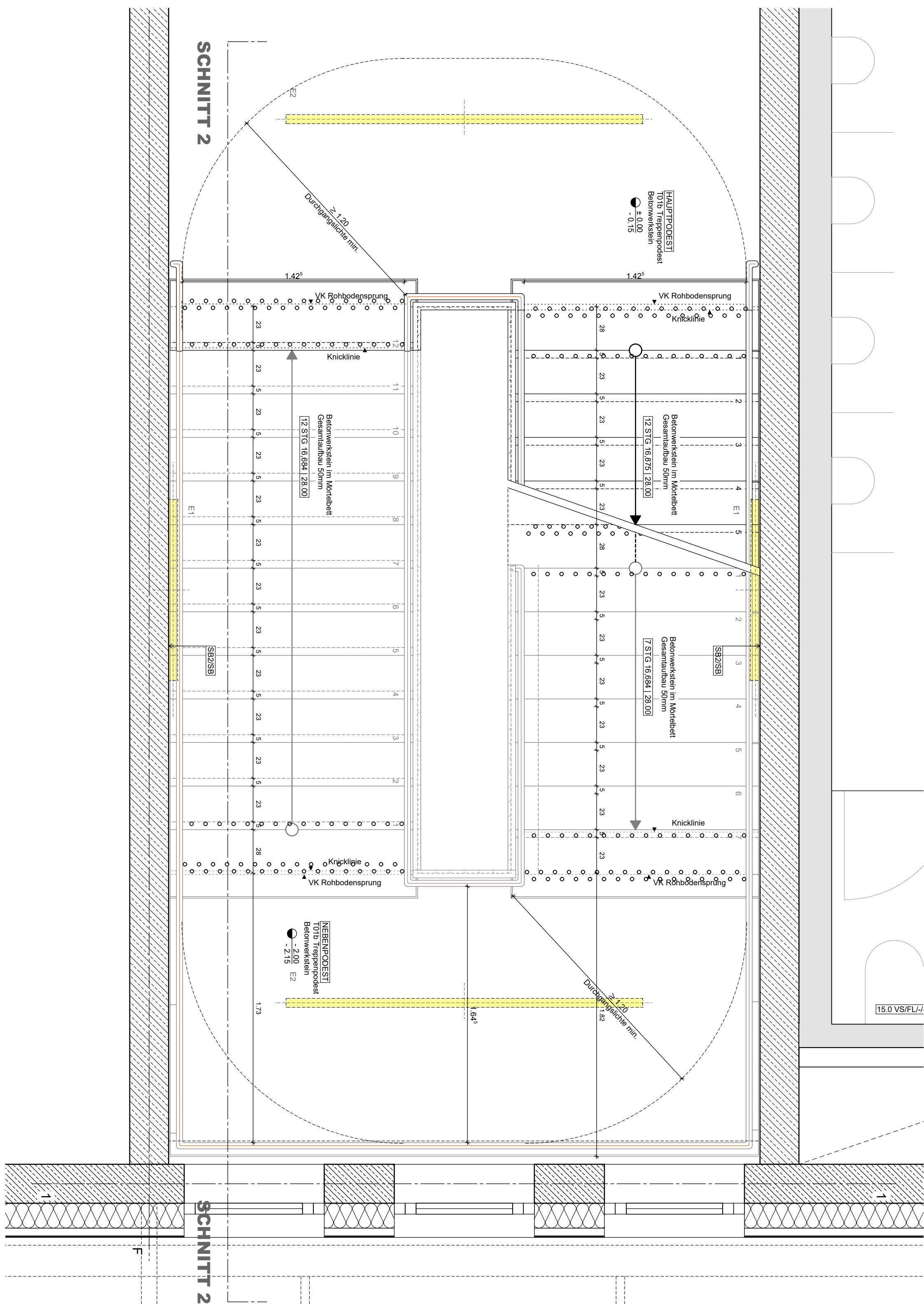
Grundriss EG
