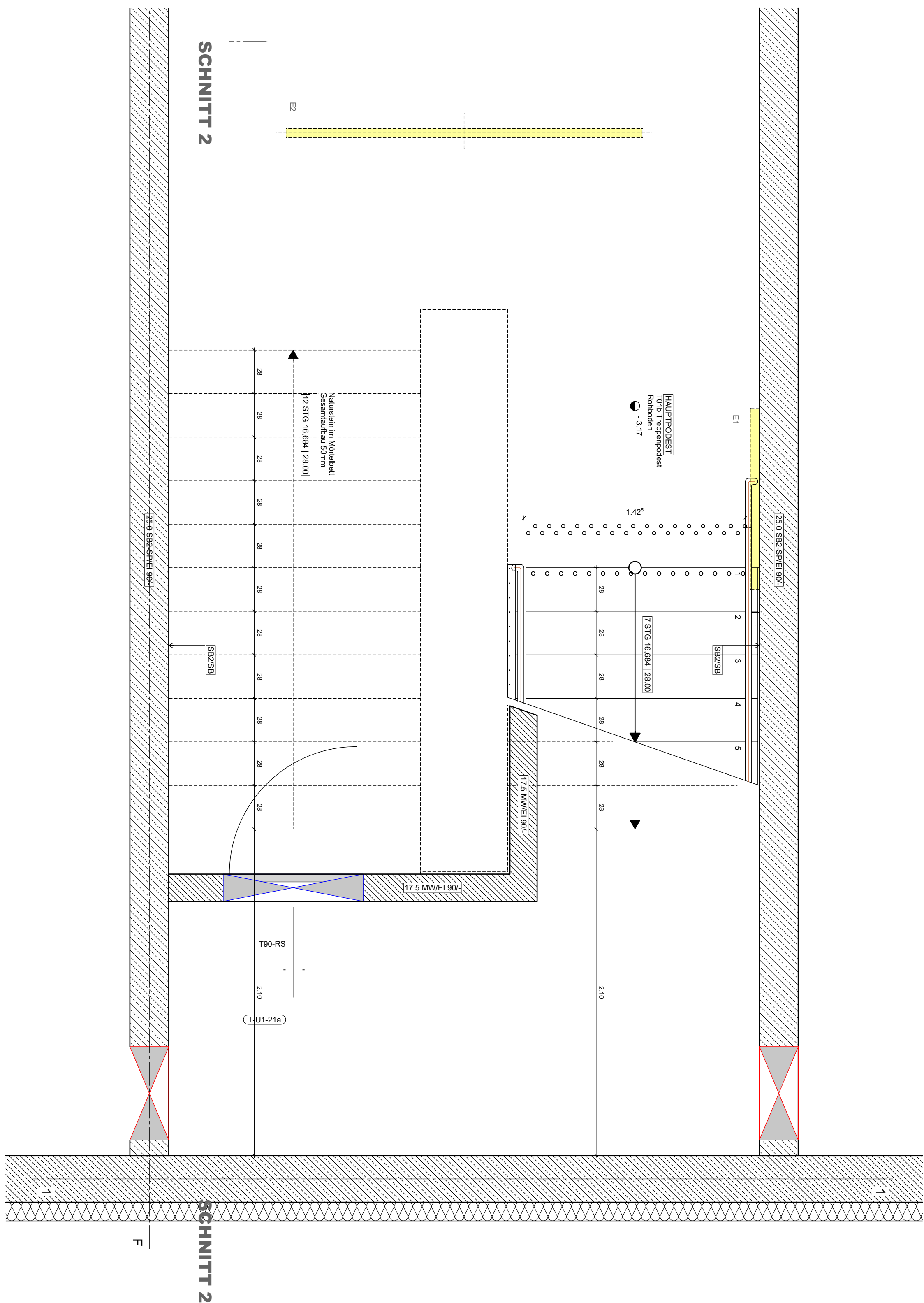
Grundriss UG
