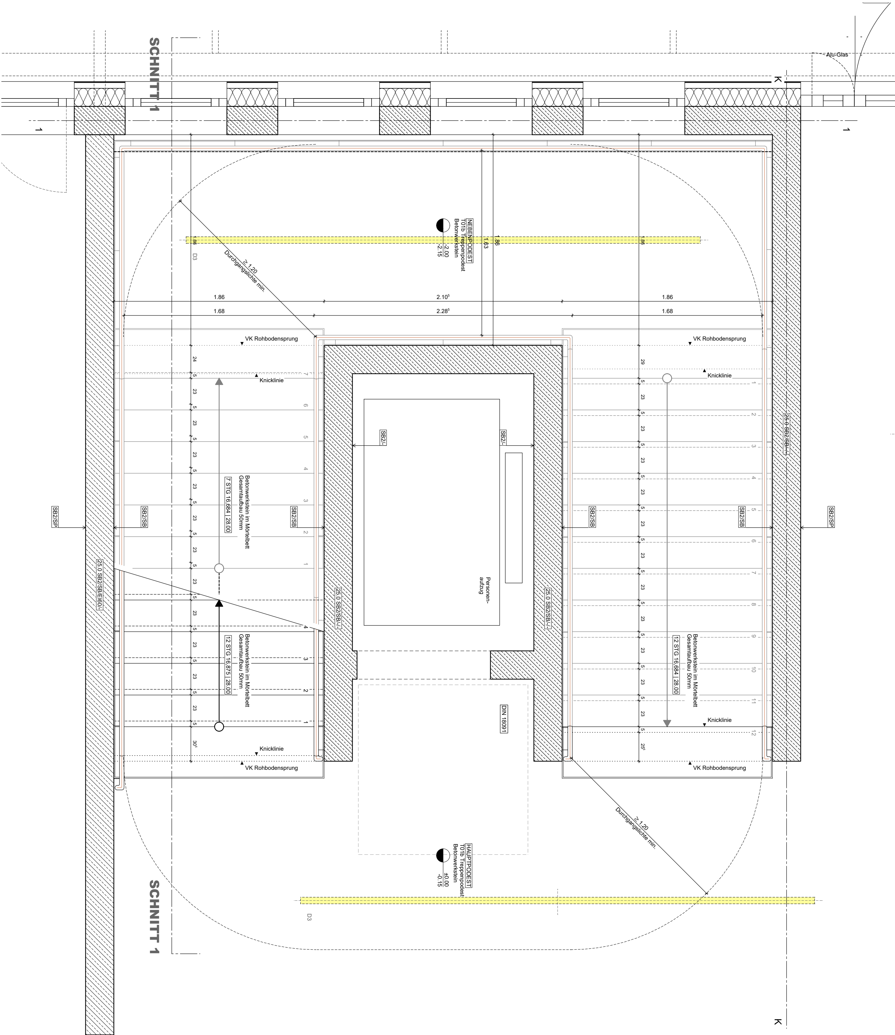
Grundriss EG
