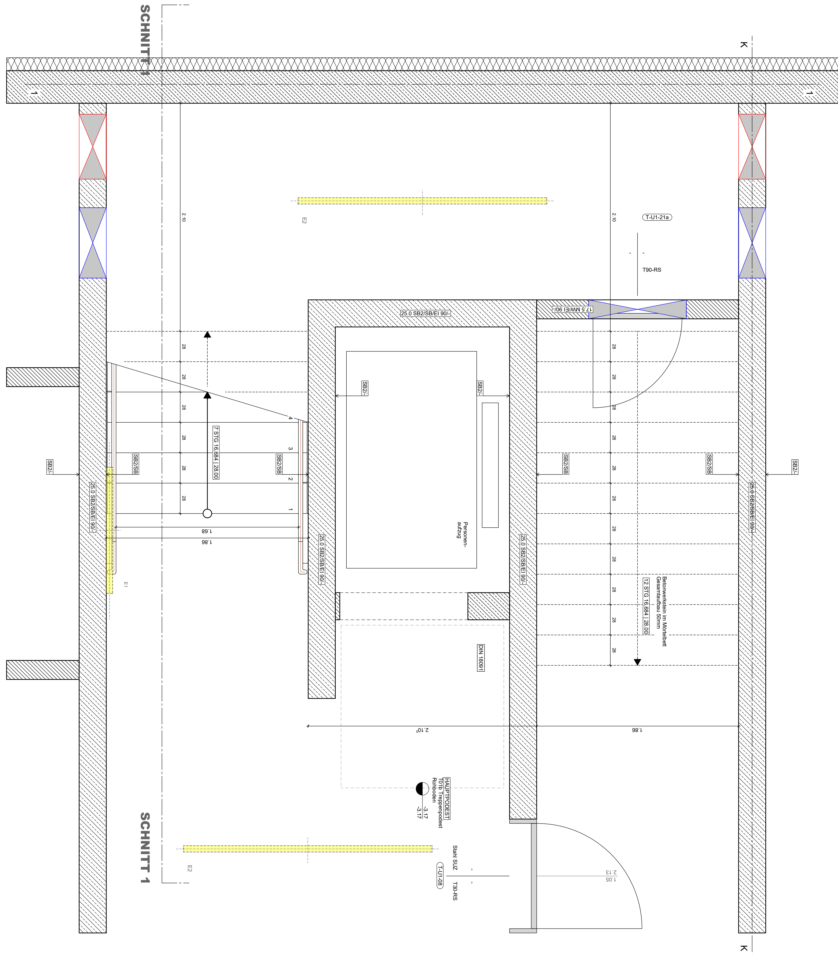
Grundriss UG
