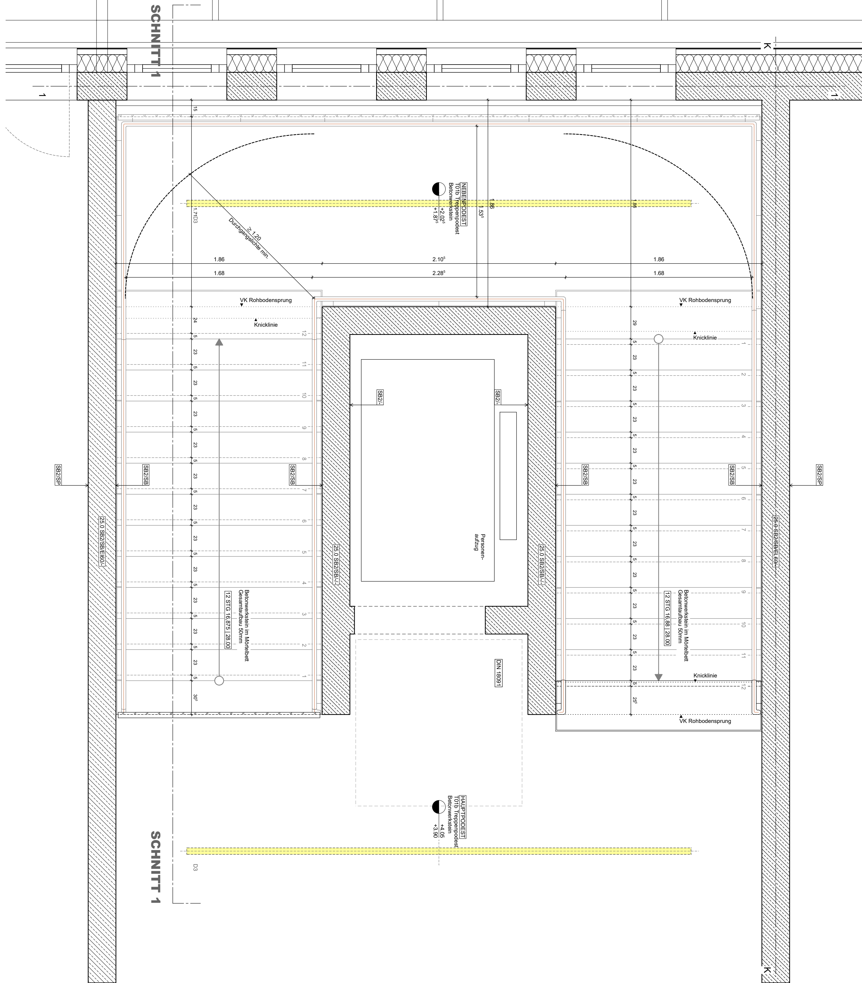
Grundriss OG
