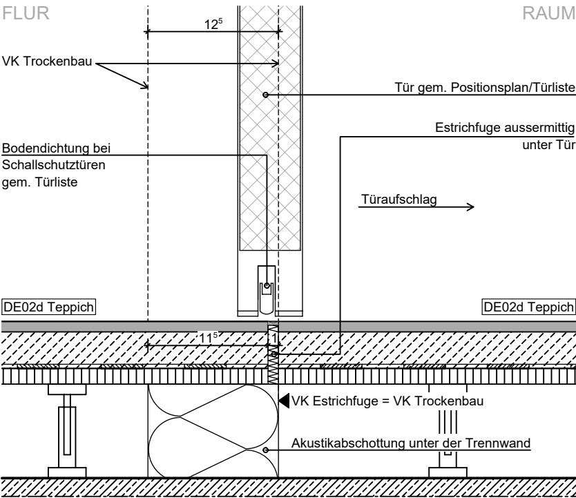
10 Anschluss Tür HUZ - DE02
