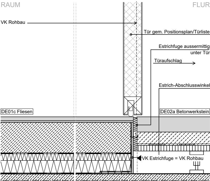
7 Anschluss Tür SDfz - DE02/DE01
