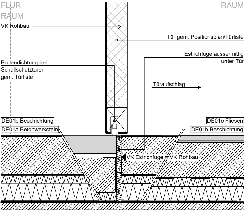
1 Anschluss Tür SUz - DE01
