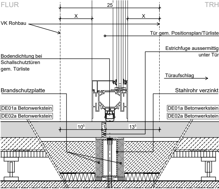
4 Anschluss Tür MRG - DE01/DE02
