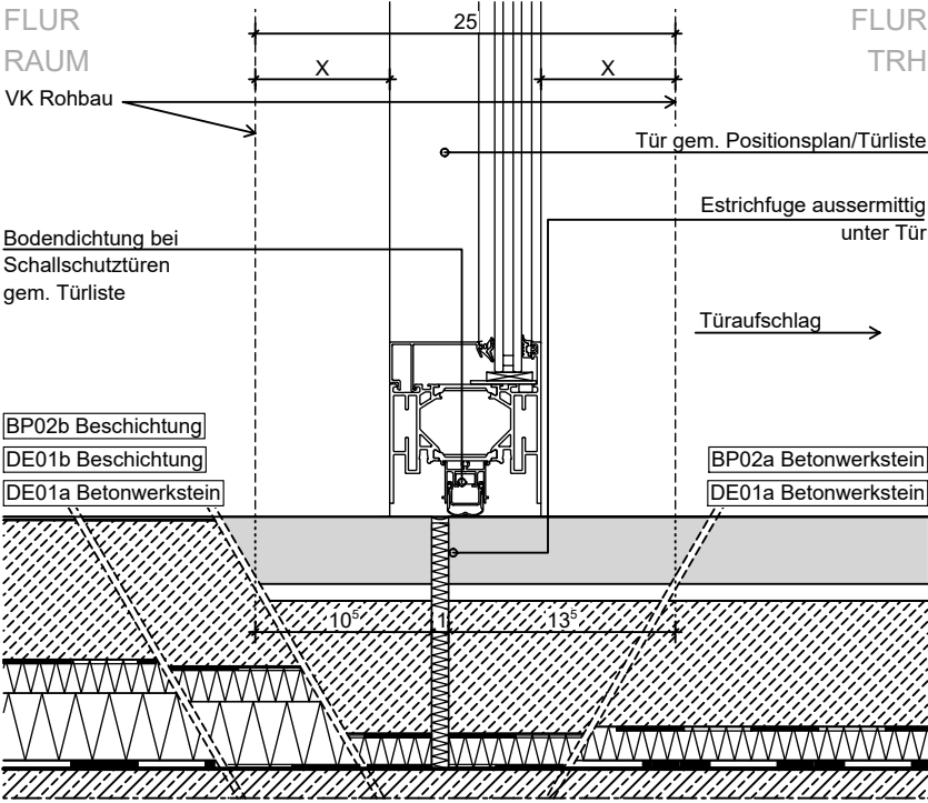
2 Anschluss Tür MRG - DE01/BP02
