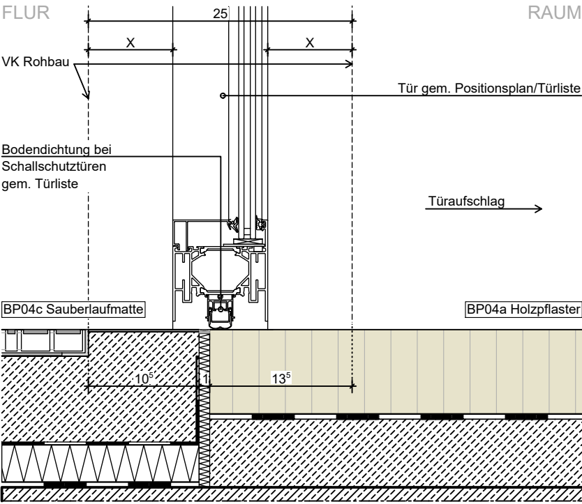
3 Anschluss Tür MRG - BP04
