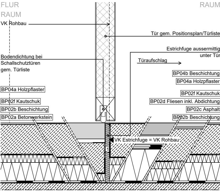
1 Anschluss Tür SUz - BP02/BP04
