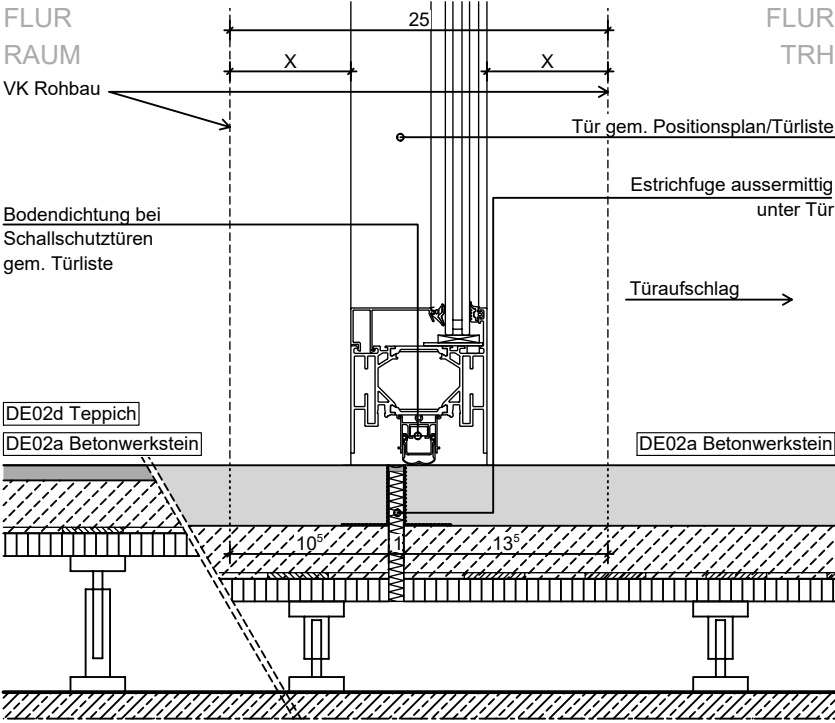
2 Anschluss Tür MRG - DE02
