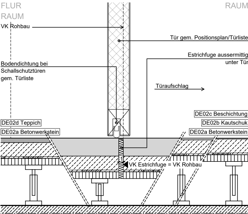
5 Anschluss Tür SUz - DE02
