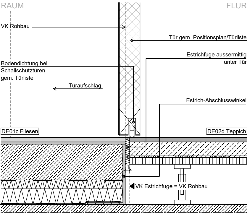
6 Anschluss Tür SUz - DE02/DE01
