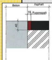
M VaB 2013 Bild A 2.5: Detail - Pressfuge
