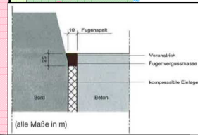
M VaB 2013 Bild A 2.5: Detail - Raumfuge
