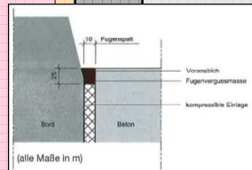
M VaB 2013 Bild A 2.5: Detail - Raumfuge
