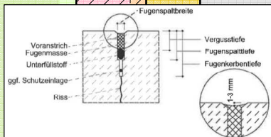
ZTV Fug-StB 15 Bild 1: Querschnitt in Fahrbahndecken aus Beton
