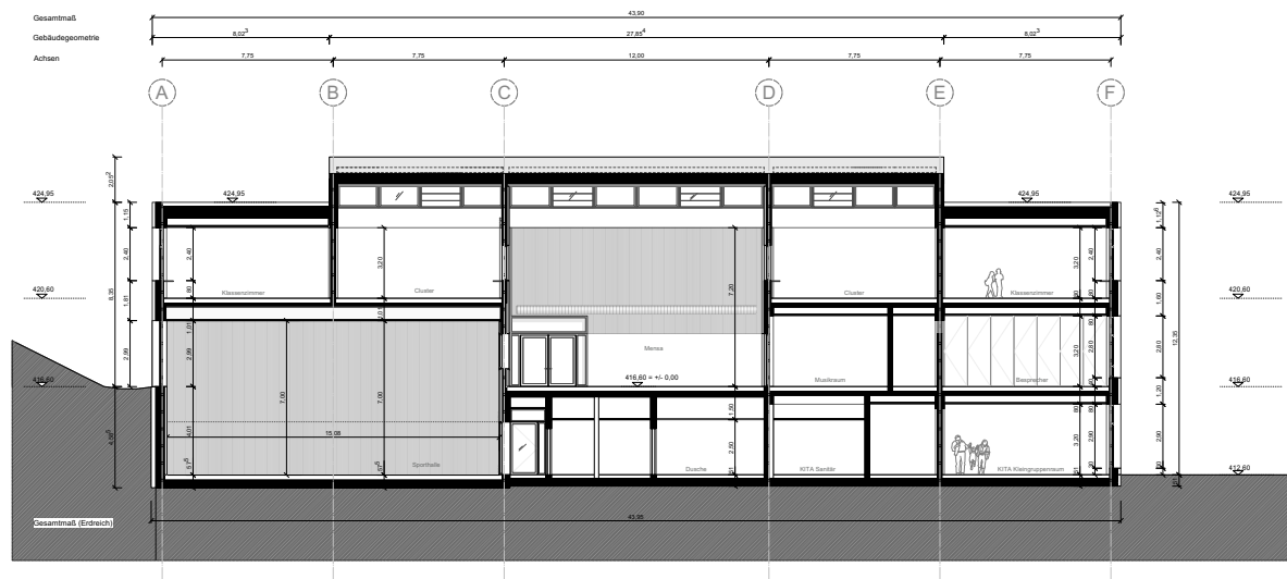
Schnitt A-A' M 1:100
