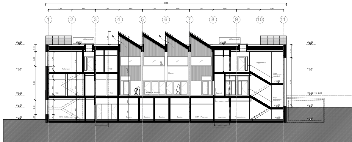
Schnitt B-B' M 1:100
