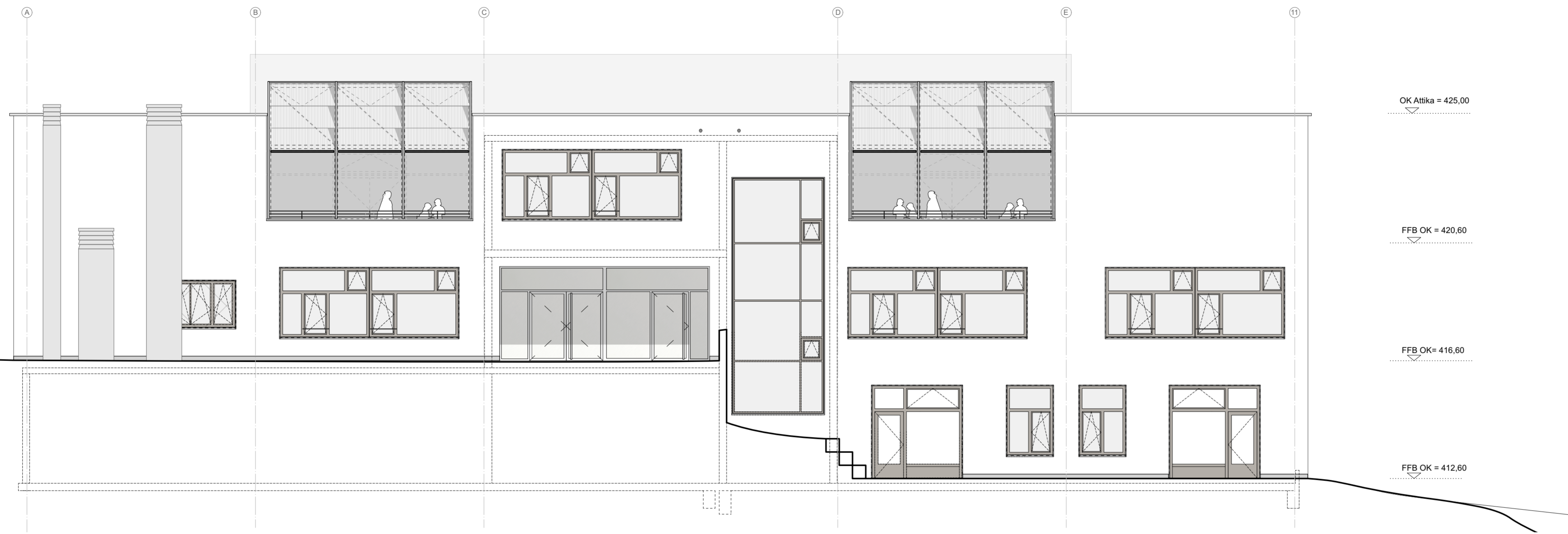
Ansicht Süd M 1:100
