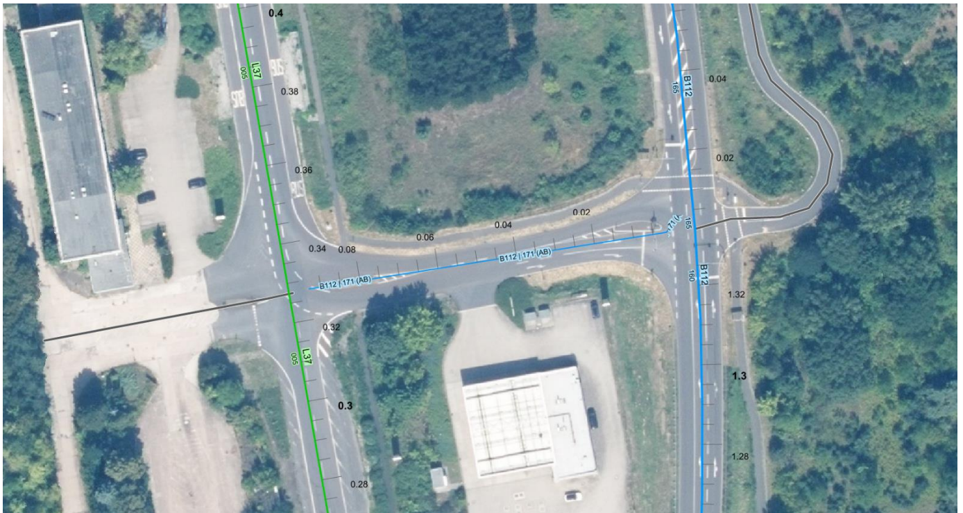
Knoten 2 Signallageplan LSA B 112 Abs 171 / L 37 Abs 005 Eisenhüttenstadt An der Pohlitzer Mühle
