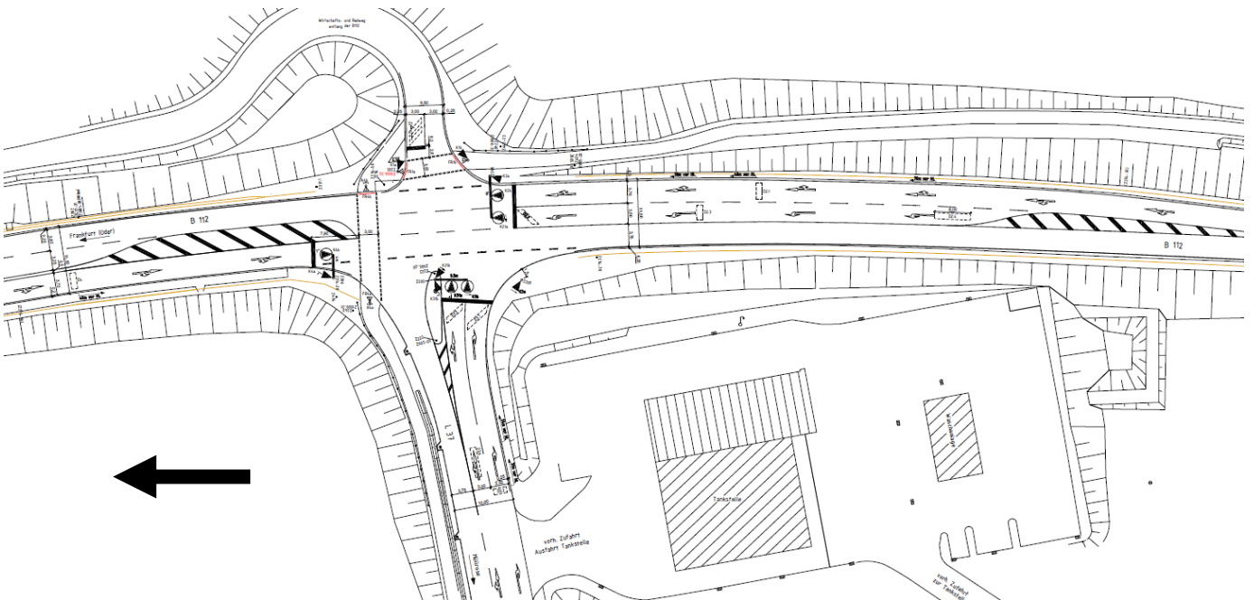
Knoten 3 B 168 Abs. 210 Fürstenwalde Lise Meitner Straße
