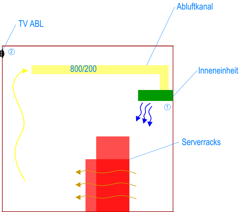
Detail Serverraum
