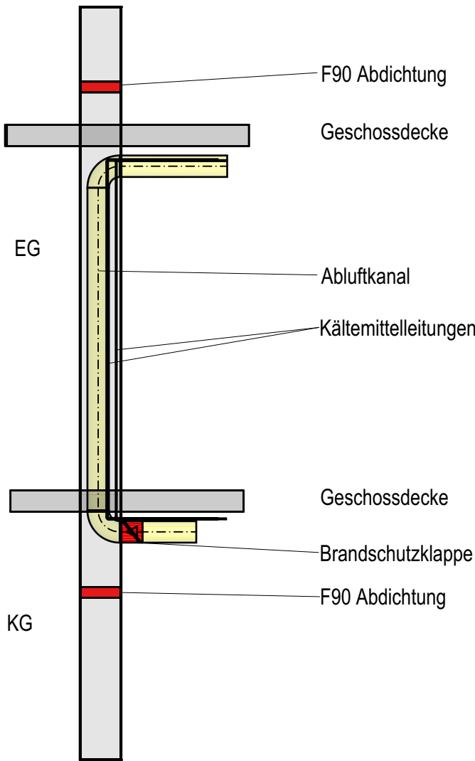
Detail Schacht 2
