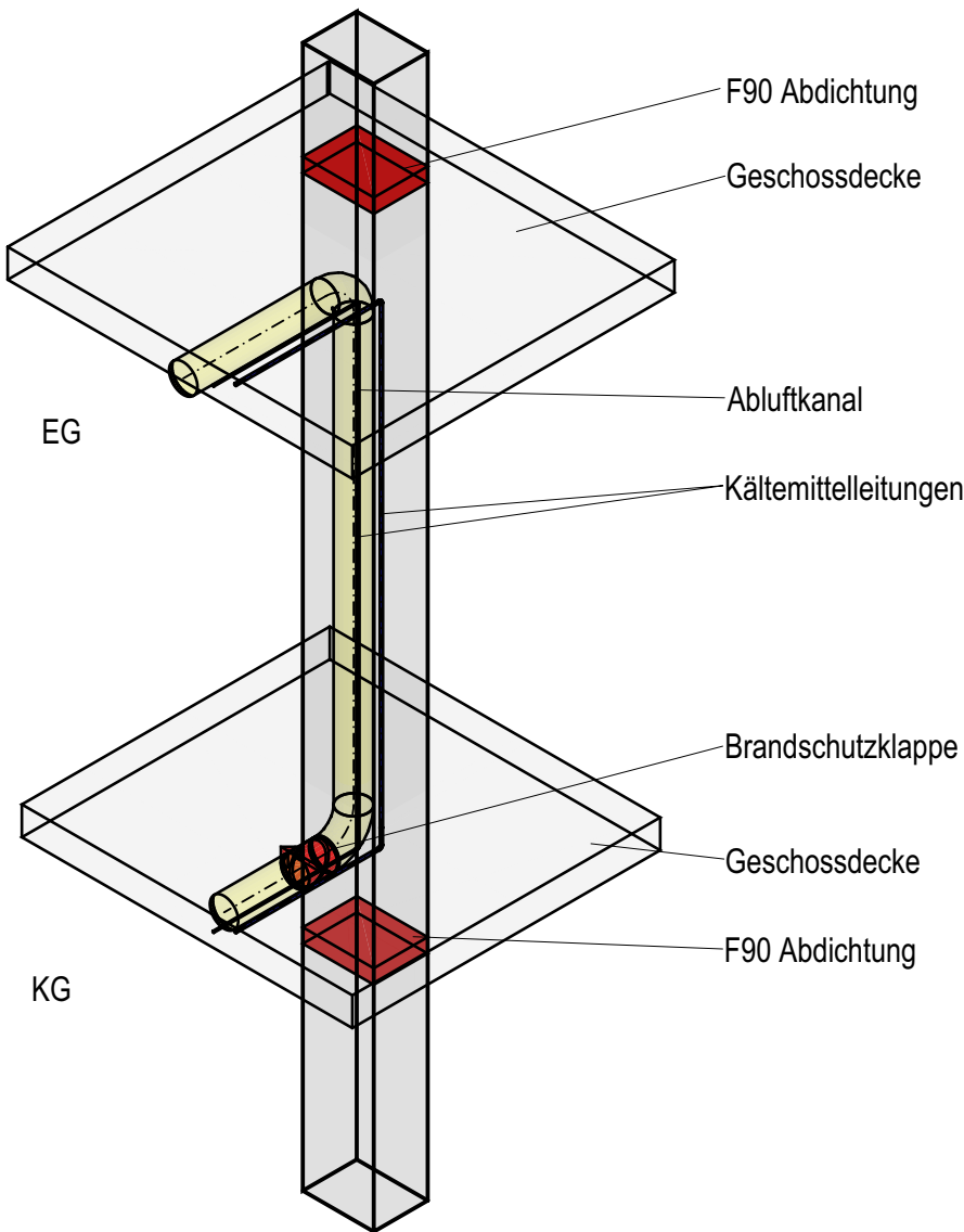
Detail Schacht 1
