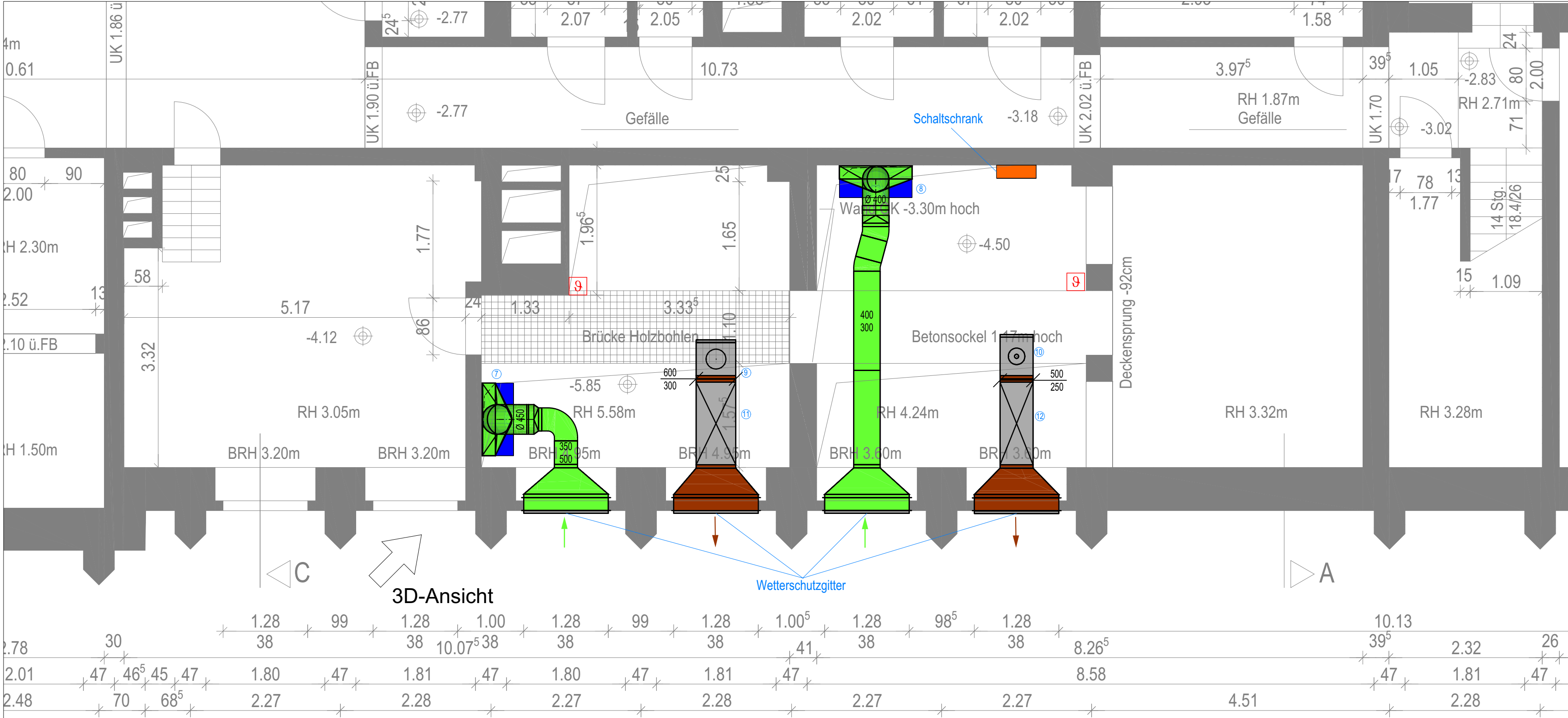
3D-Ansicht
