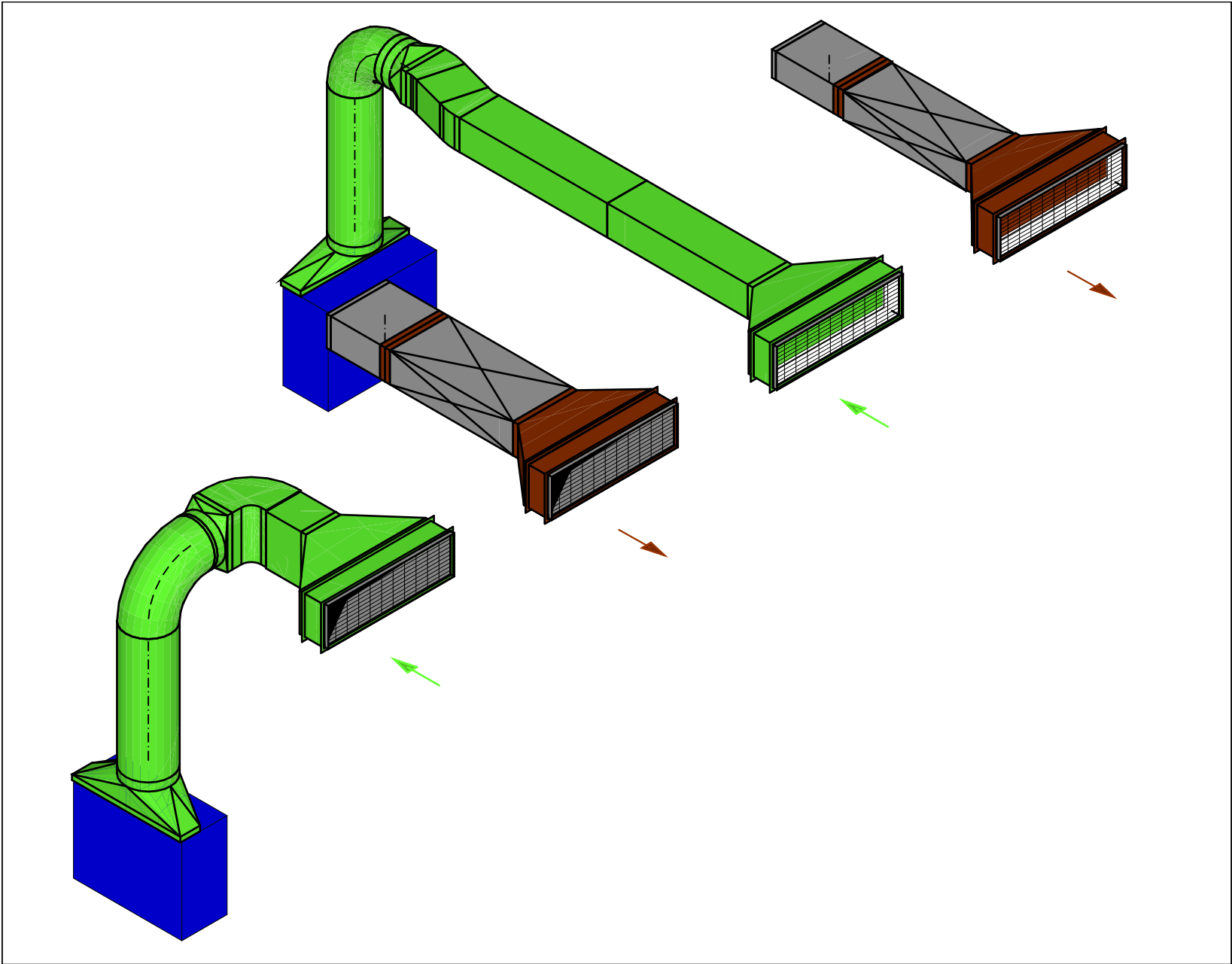
3D-Ansicht
