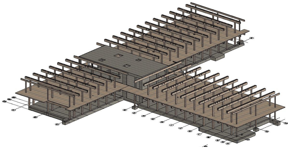
Abb. 02 Rohbau - Stahlbeton Konstruktiver Holzbau (ohne Wände und Dach)
