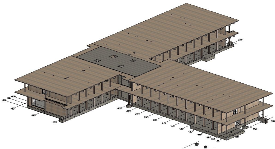
Abb. 03 Rohbau - Stahlbeton Konstruktiver Holzbau
