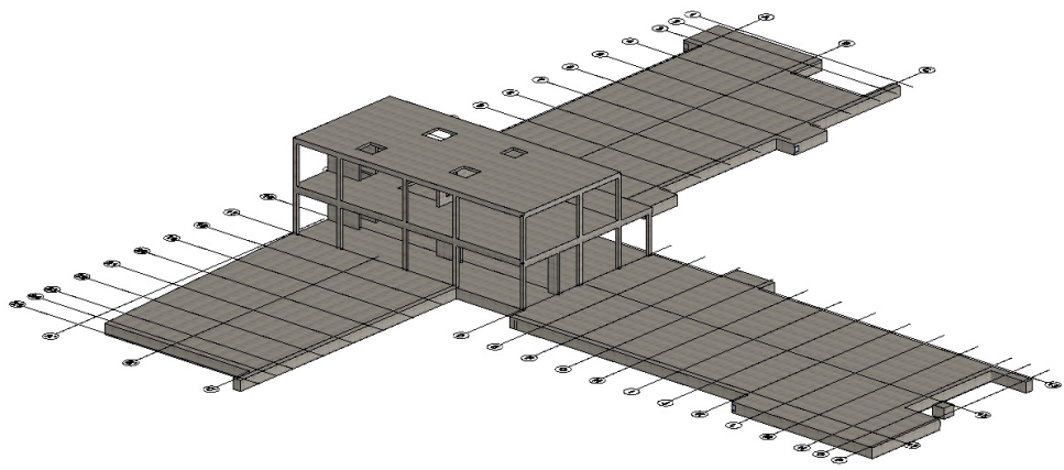
Abb. 01 Rohbau - Stahlbeton
