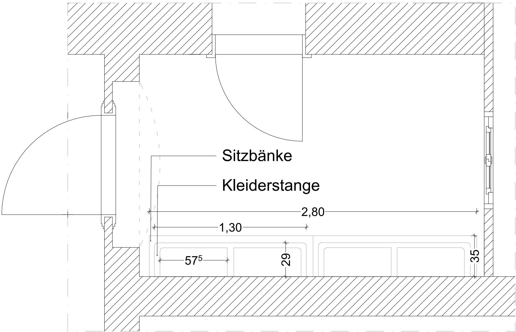
Grundriss Garderobe M 1:20
