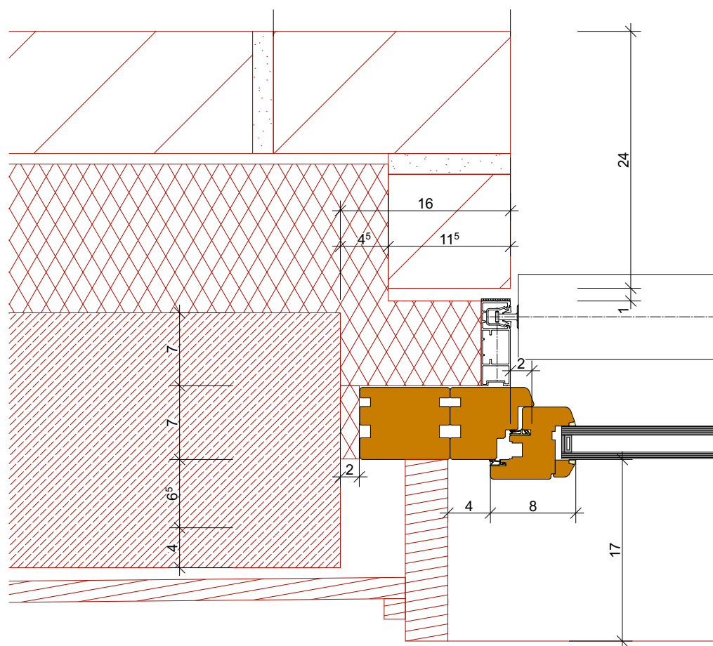
Horizontalschnitt Südseite
