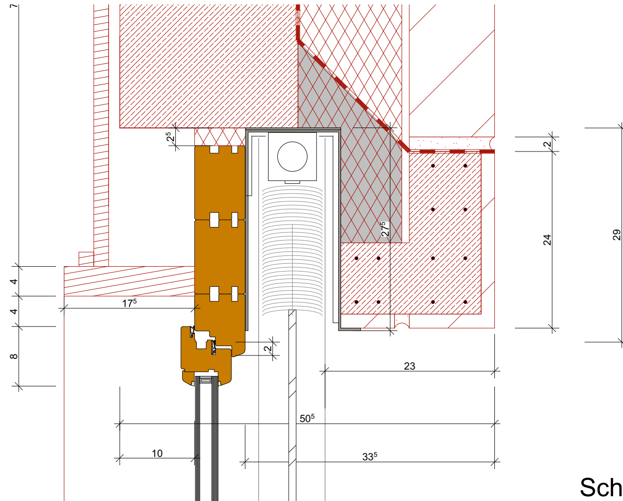
Schnitt OG Nordseite
