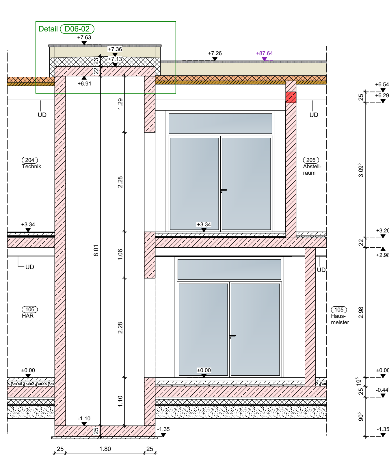
Schnitt D-D M 1:50
