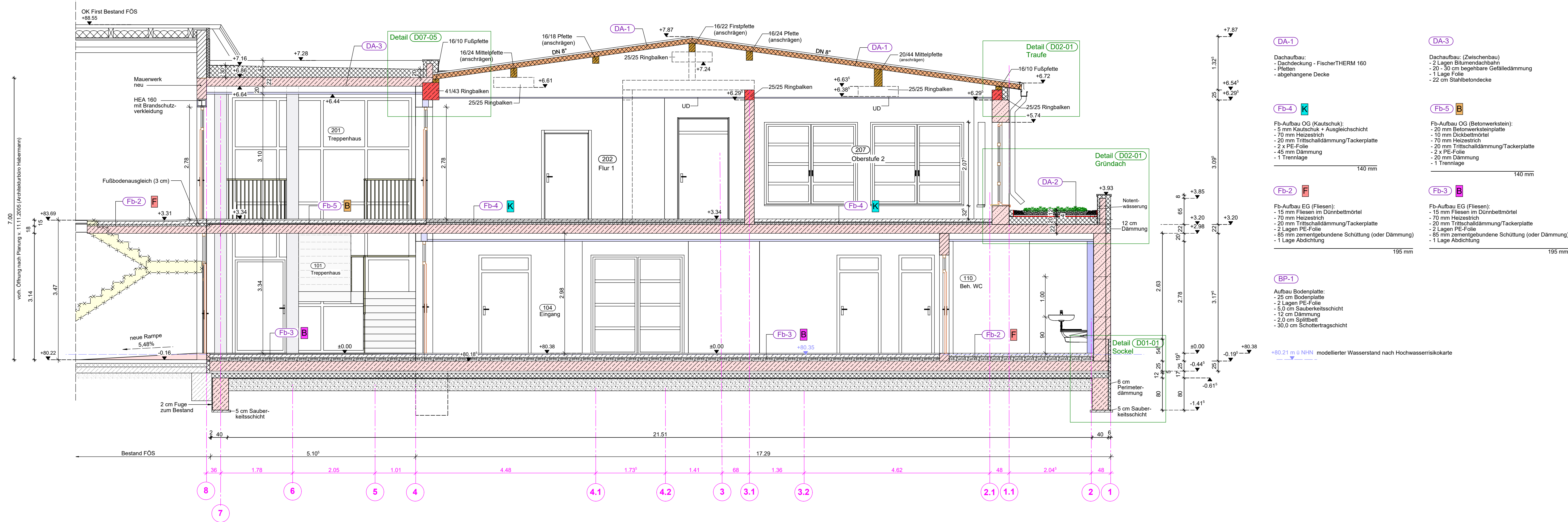
Schnitt B-B M 1:50
