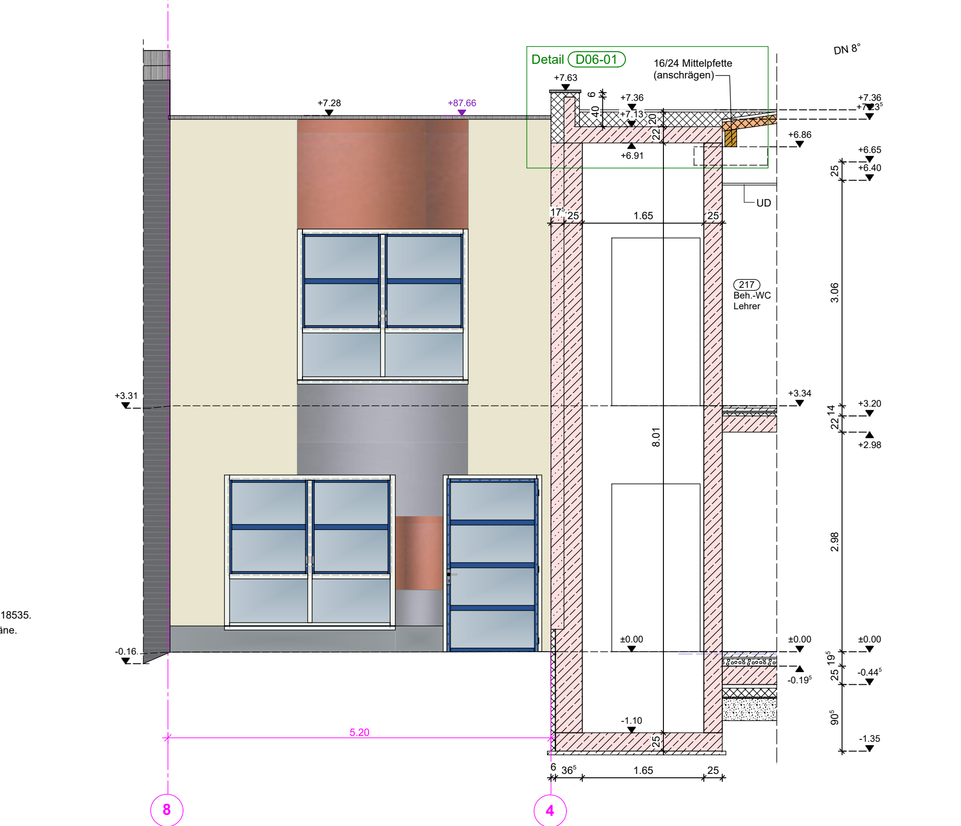
Schnitt C-C M 1:50
