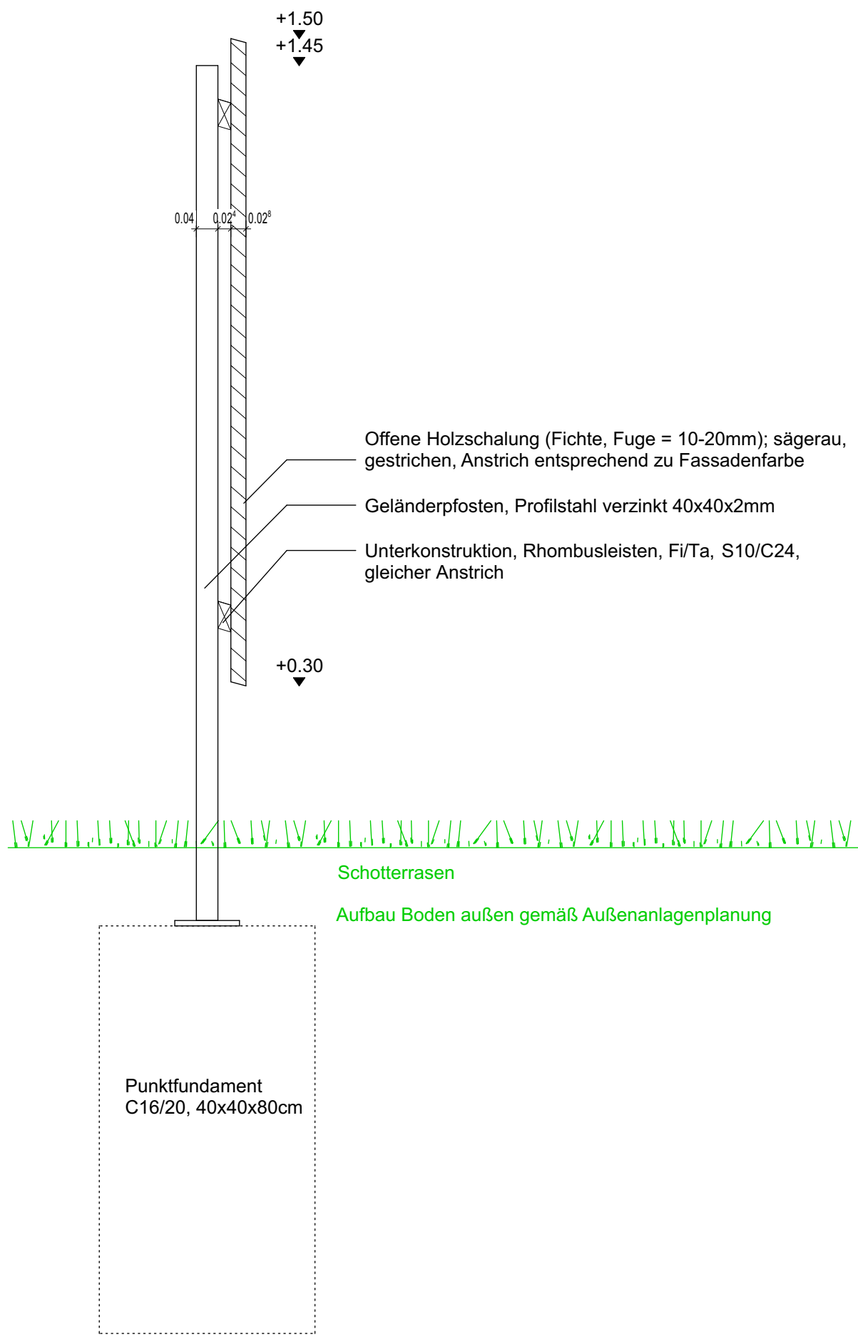
Schnitt a-a
