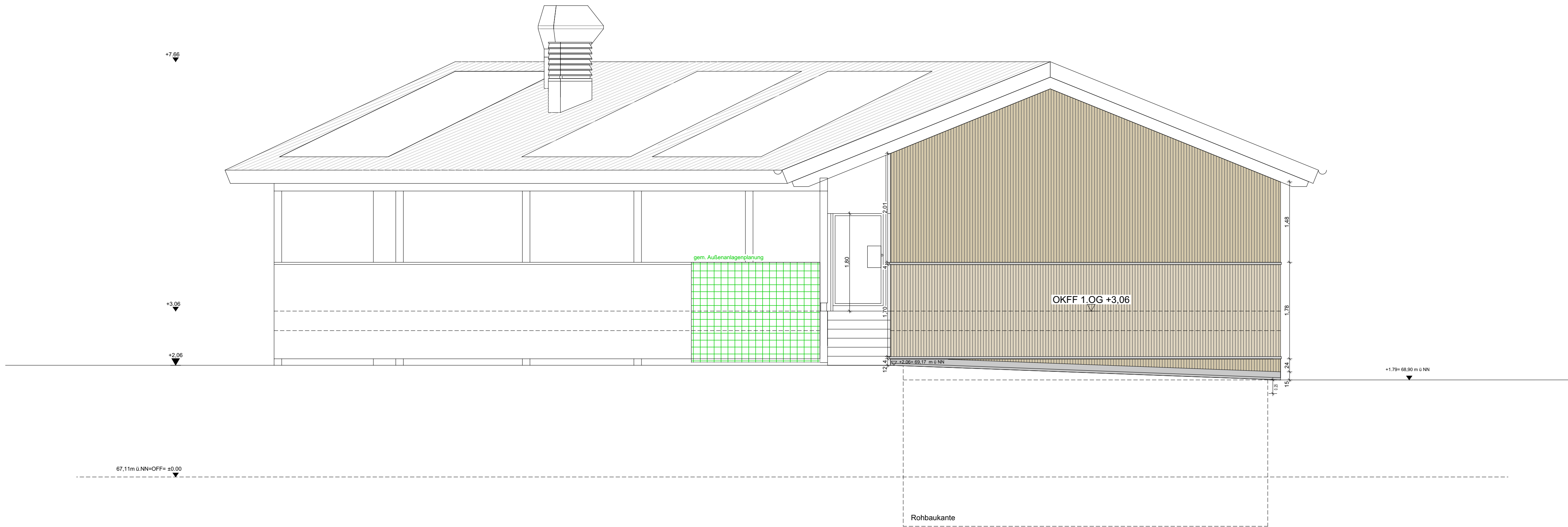
Ansicht Ost
