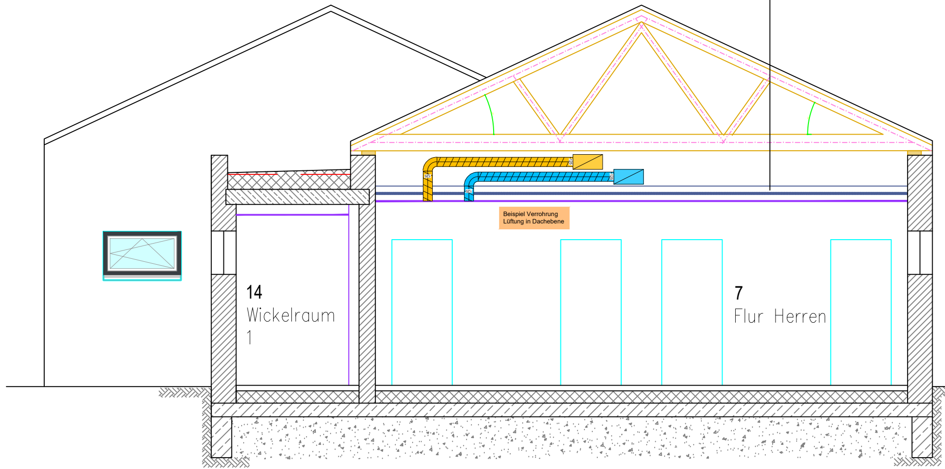
Schnitt A-A
