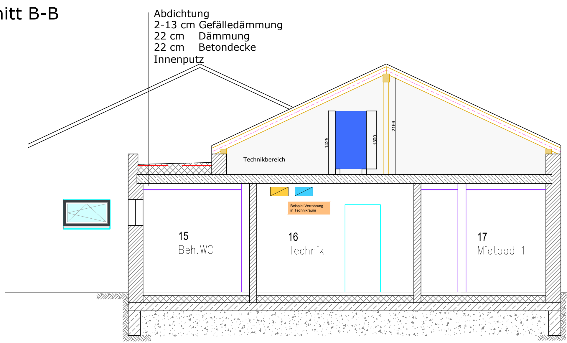
Schnitt B-B
