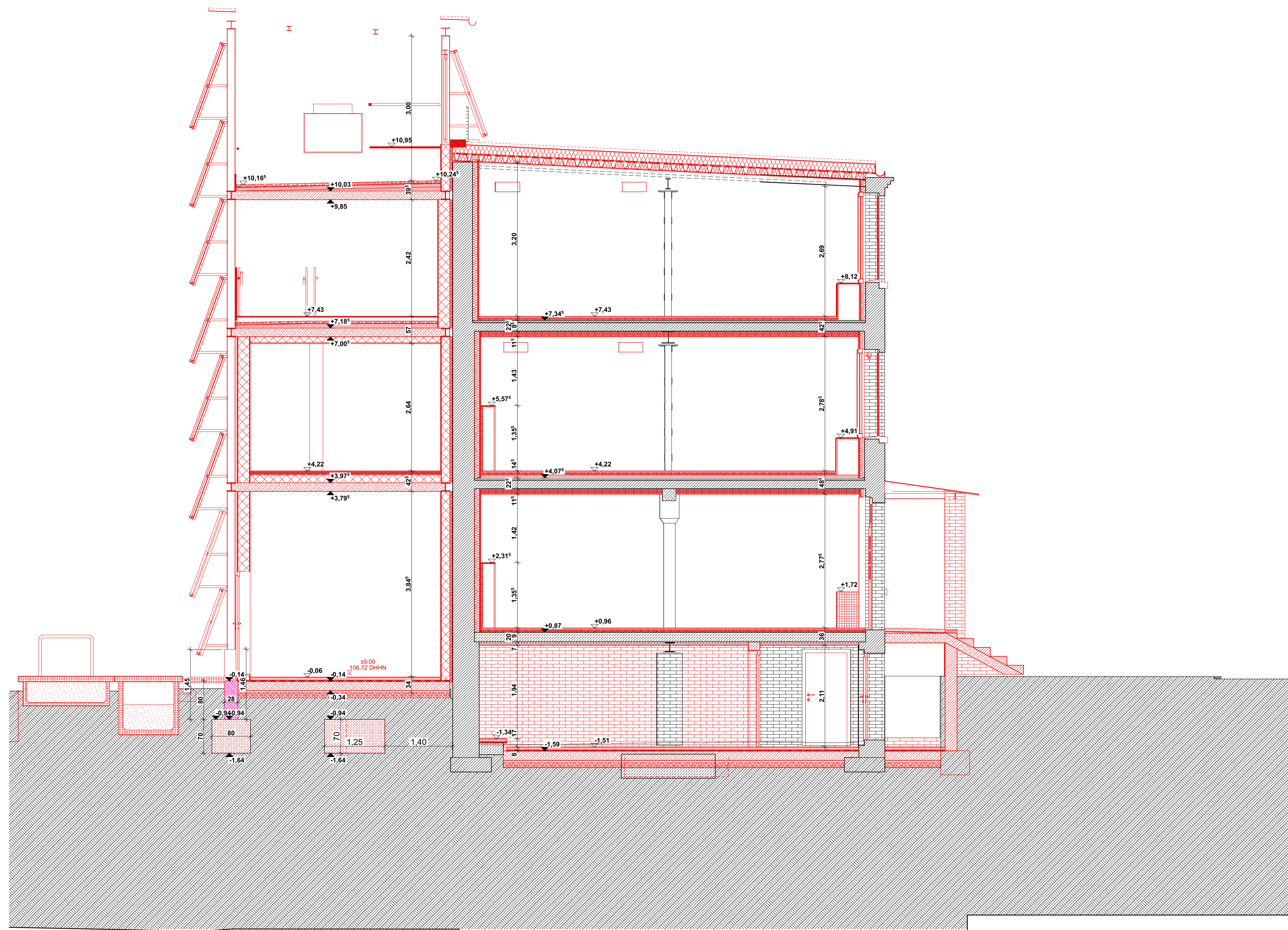
Querschnitt 2
