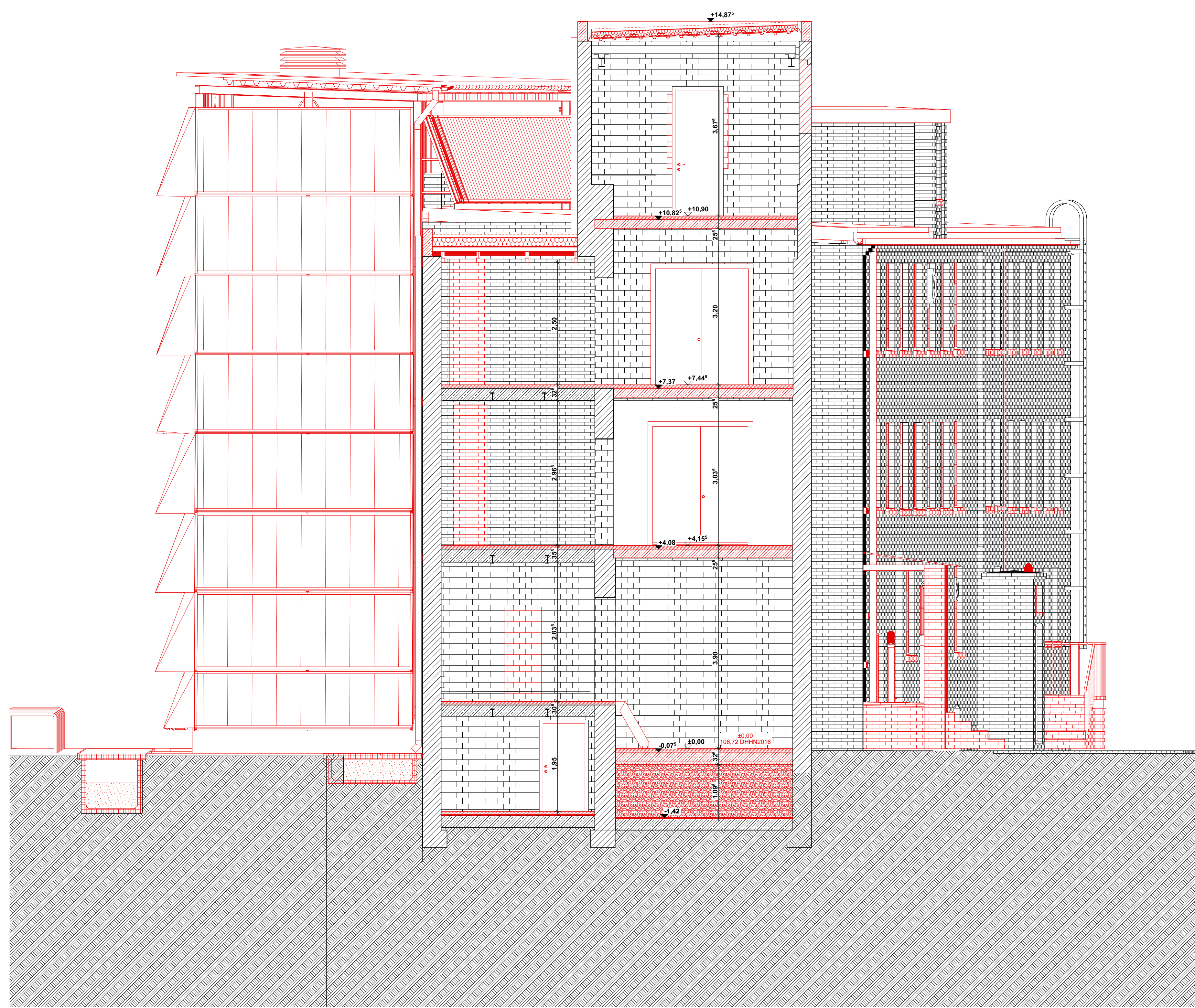
Querschnitt 1
