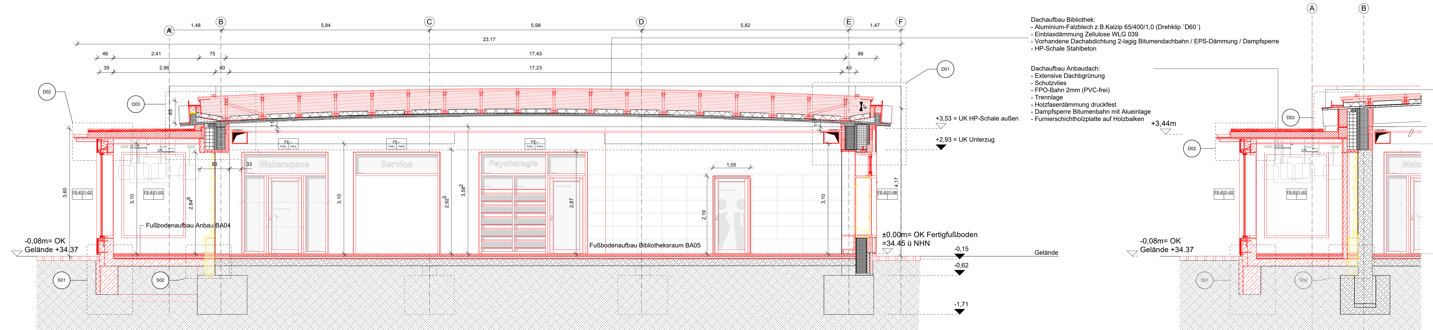
Schnitt B-B
