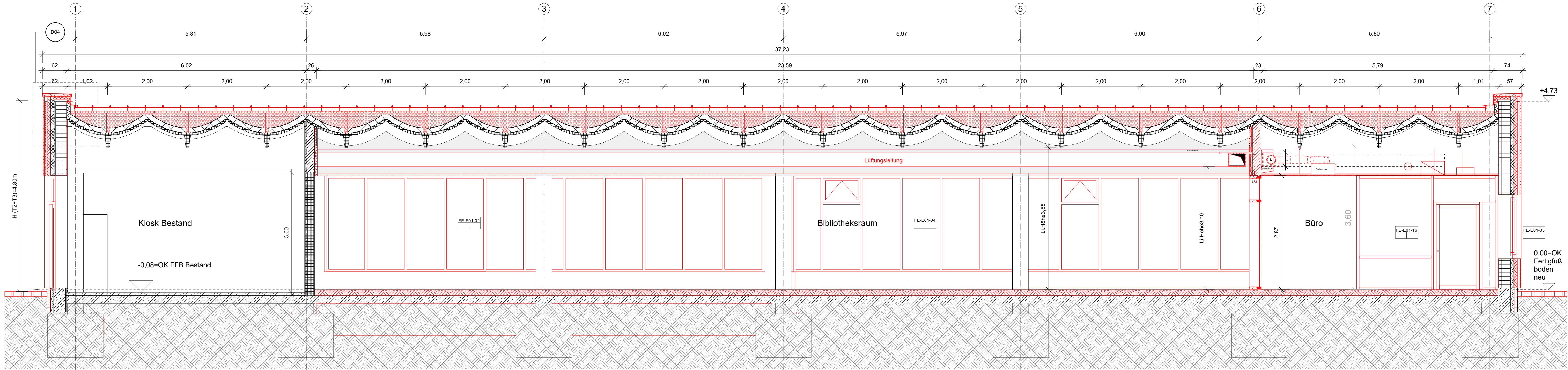
Schnitt A-A
