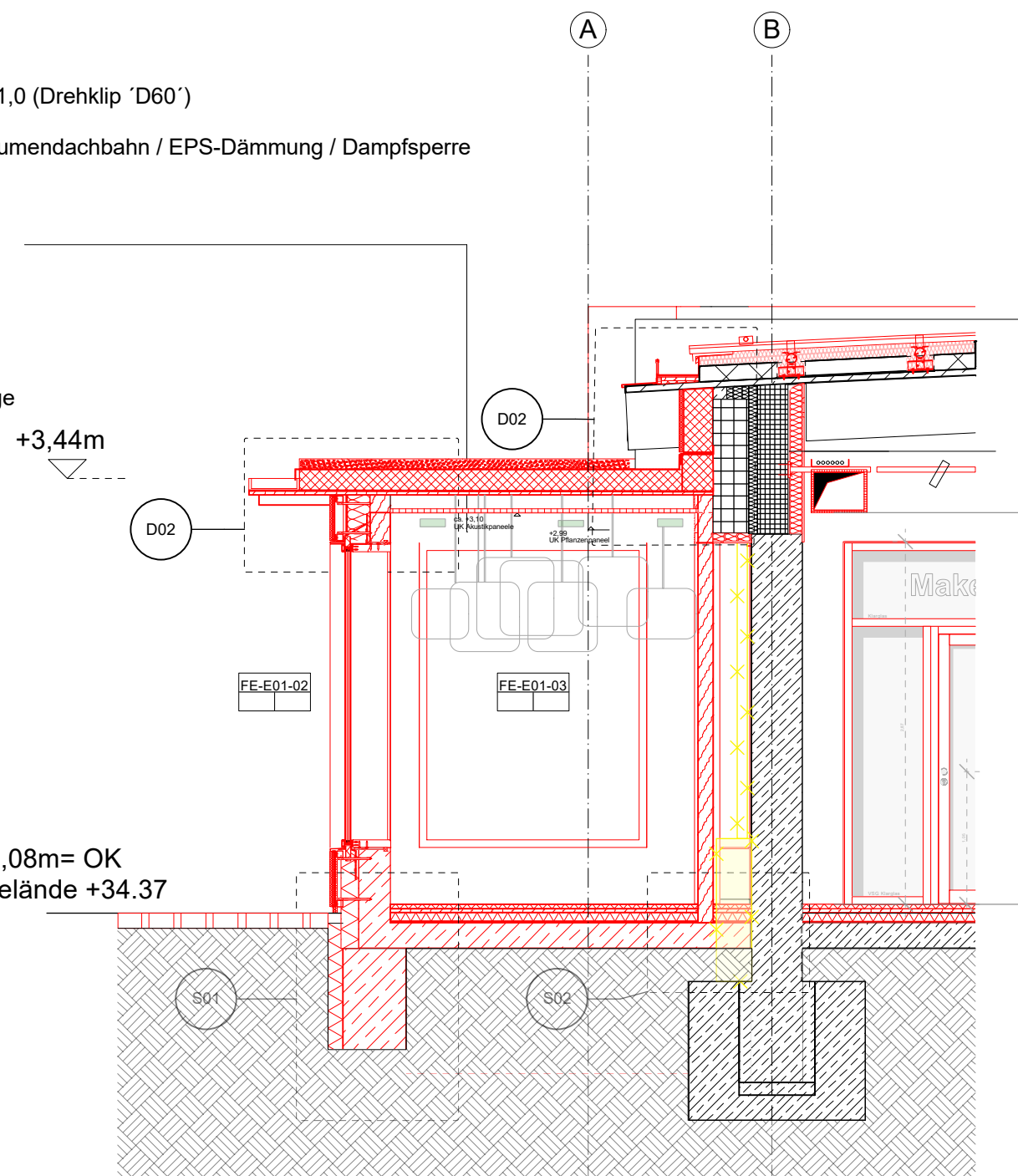
Schnitt C-C
