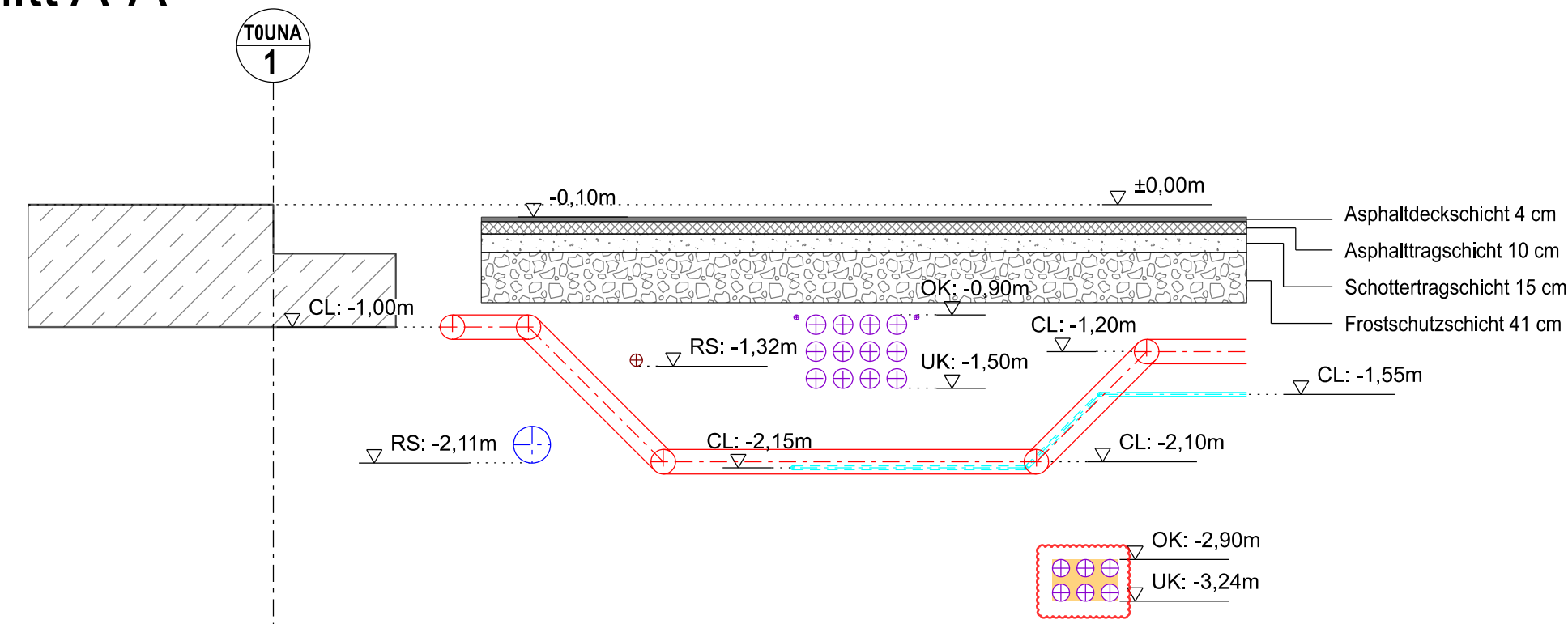
Schnitt A-A
