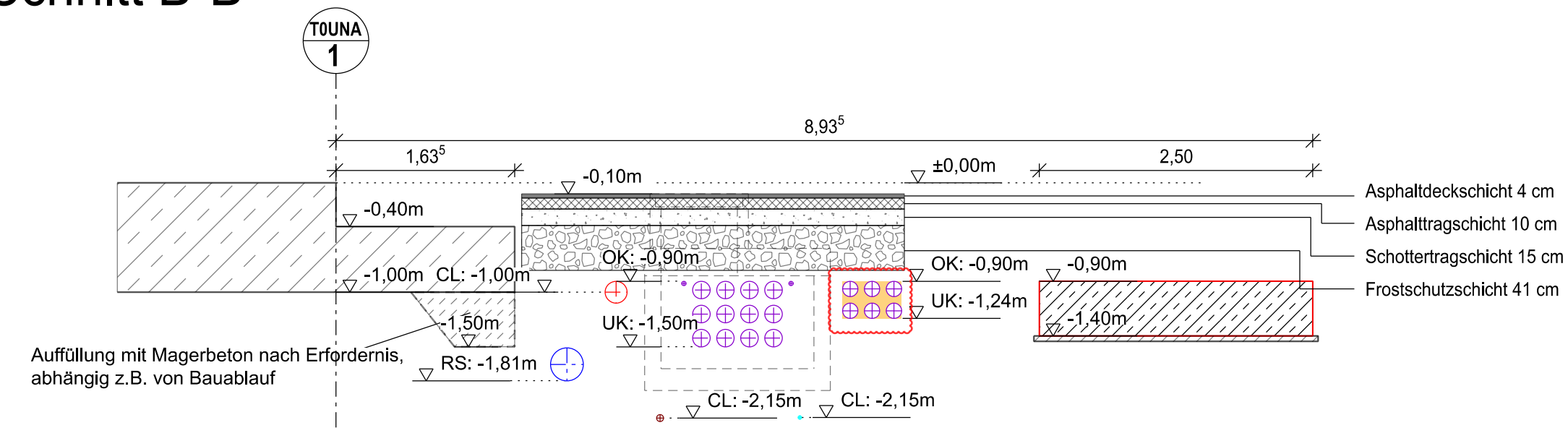
Schnitt B-B
