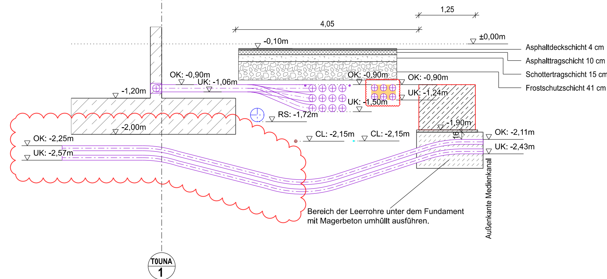
Schnitt E-E
