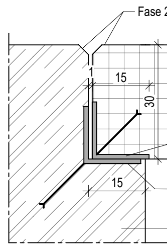
Detail Betondecke Auflager längs M 1:10
