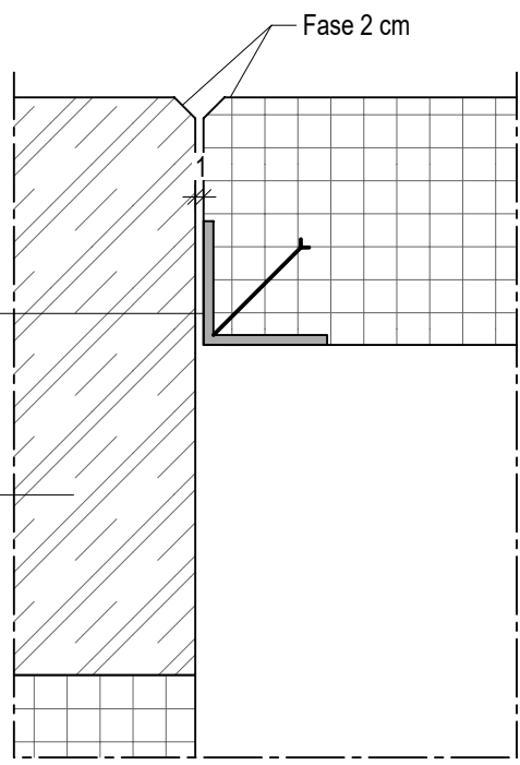
Detail Betondecke Auflager quer - befahrbar M 1:10
