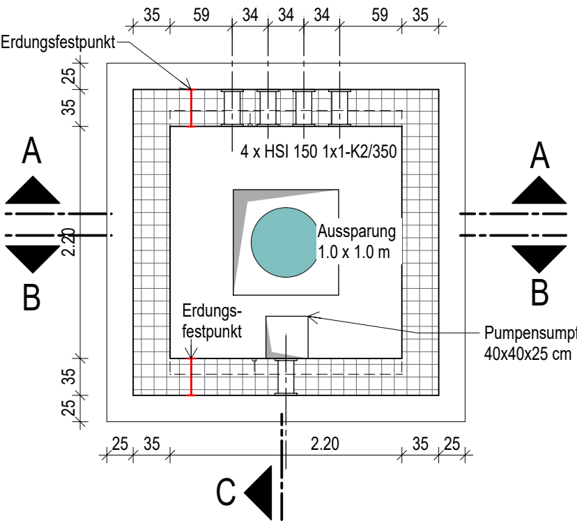
Grundriss UG M 1:50
