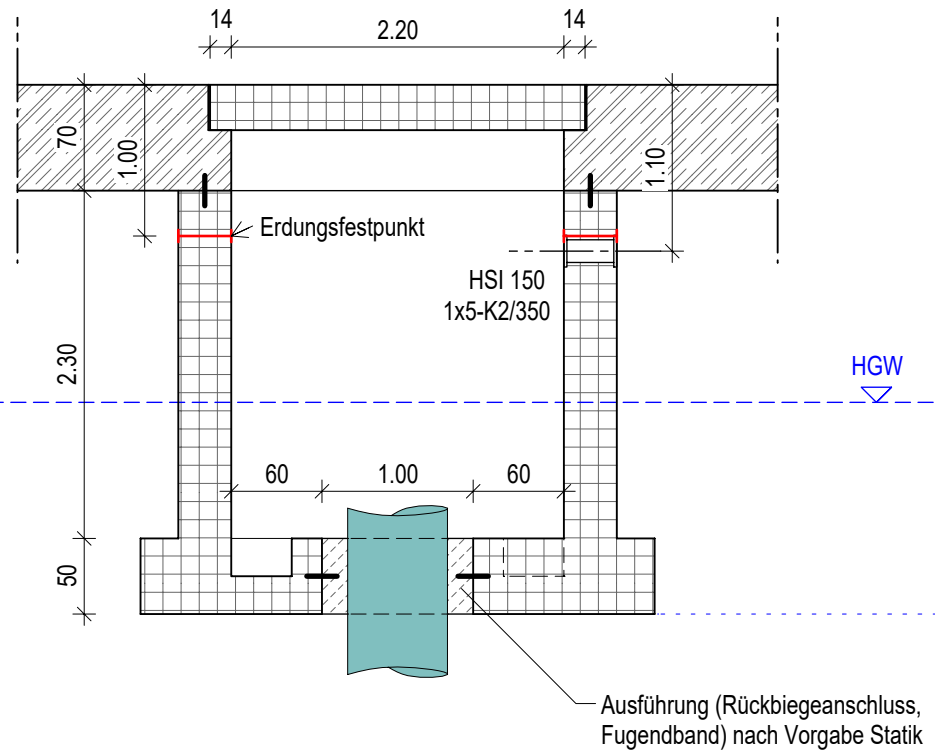
Schnitt C-C M 1:50
