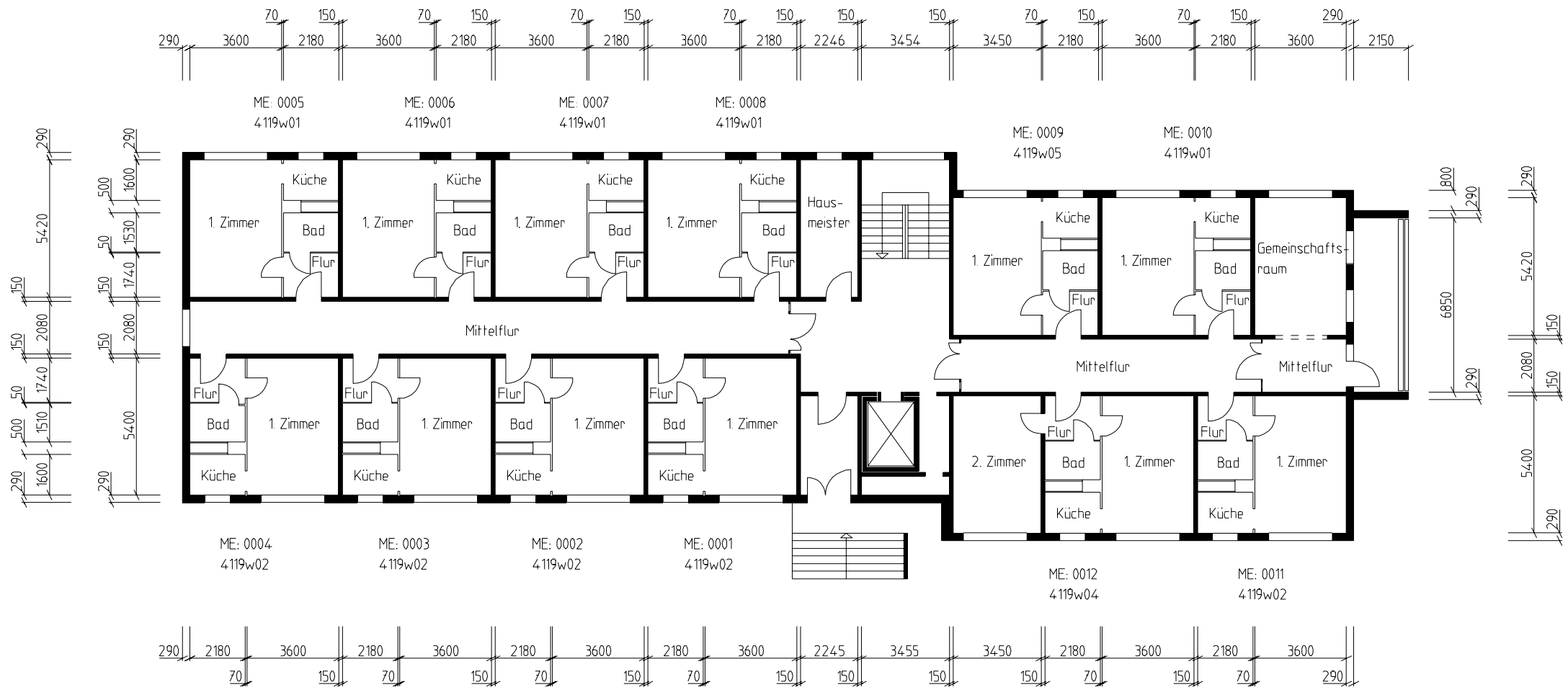
Bauweise "Altersgerechtes Wohnen", Erdgeschoß Cottbus, Hufelandstraße 13 GWC 4065-4119
