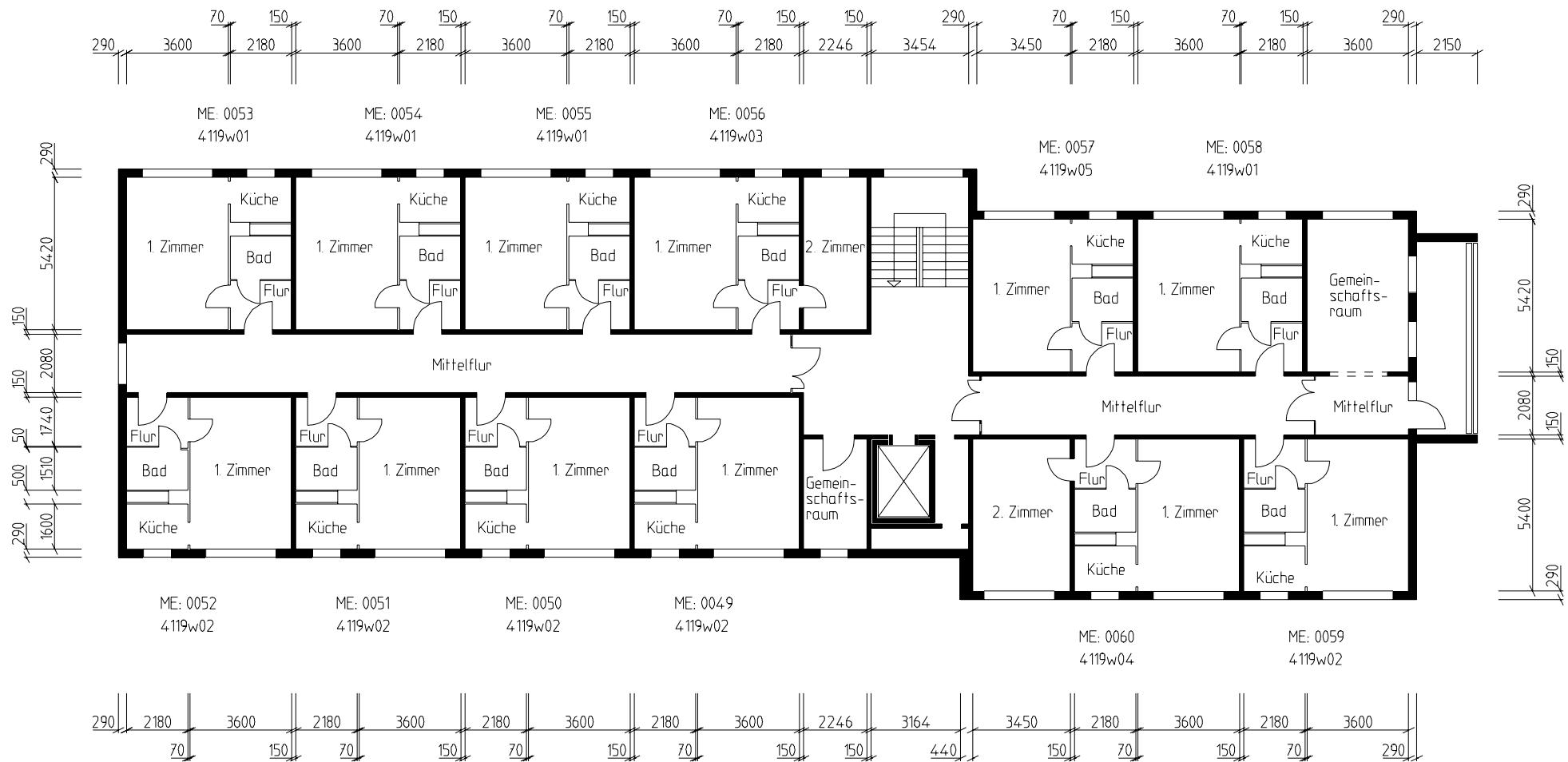
Bauweise "Altersgerechtes Wohnen", 4. Obergeschoß Cottbus, Hufelandstraße 13 GWC 4065-4119
