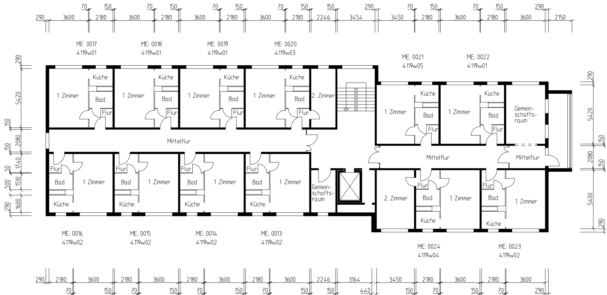
Bauweise "Altersgerechtes Wohnen", 1. Obergeschoß Cottbus, Hufelandstraße 13 GWC 4065-4119
