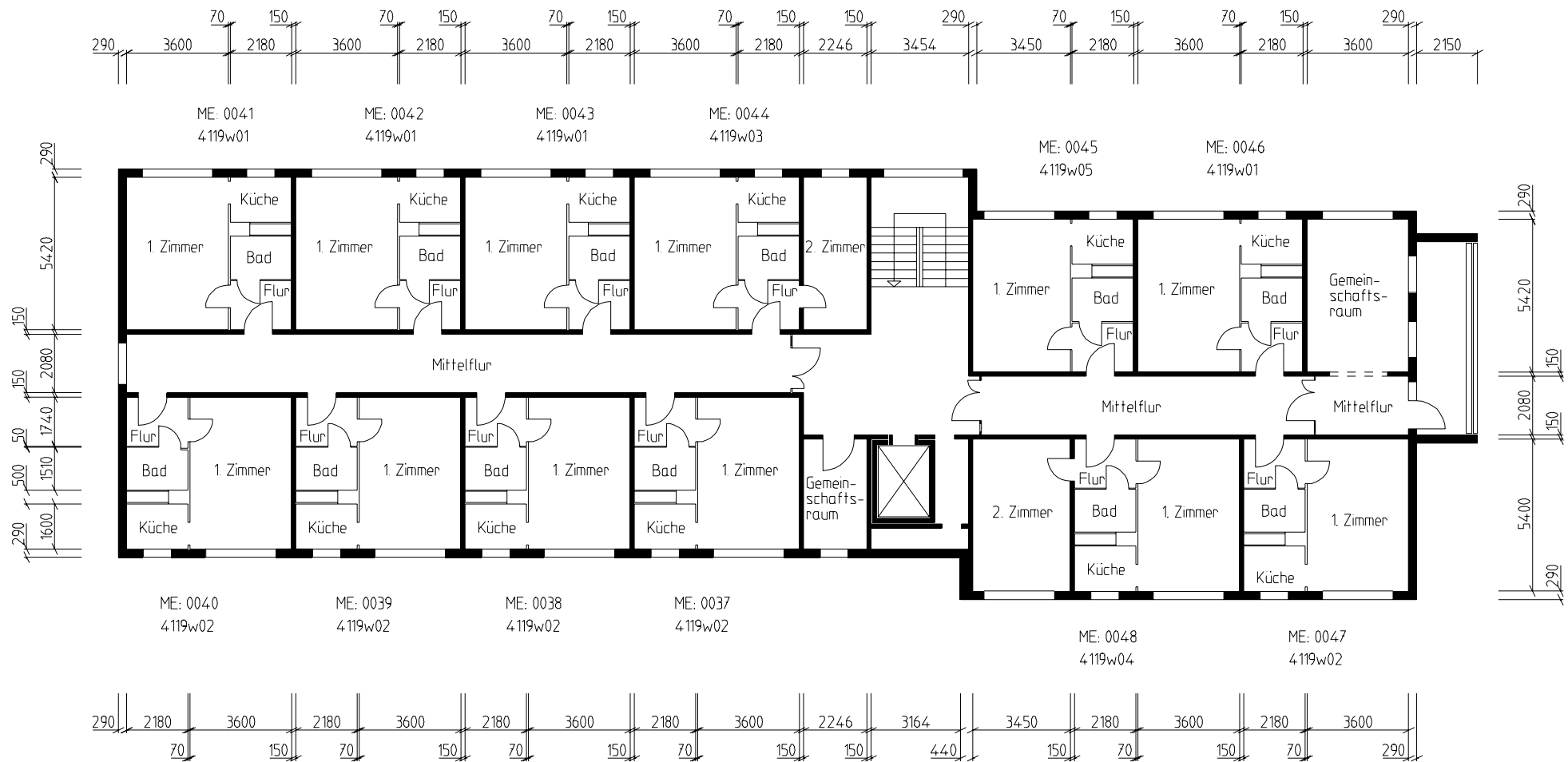
Bauweise "Altersgerechtes Wohnen", 3. Obergeschoß Cottbus, Hufelandstraße 13 GWC 4065-4119
