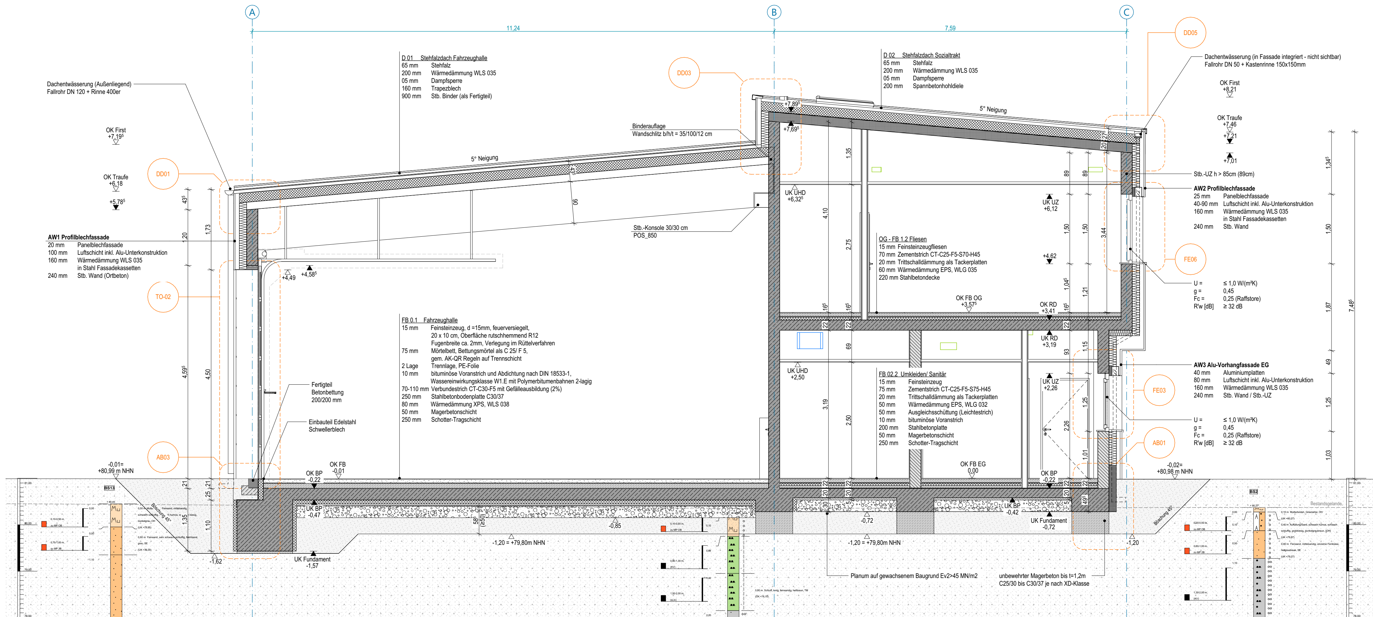
Schnitt AA
