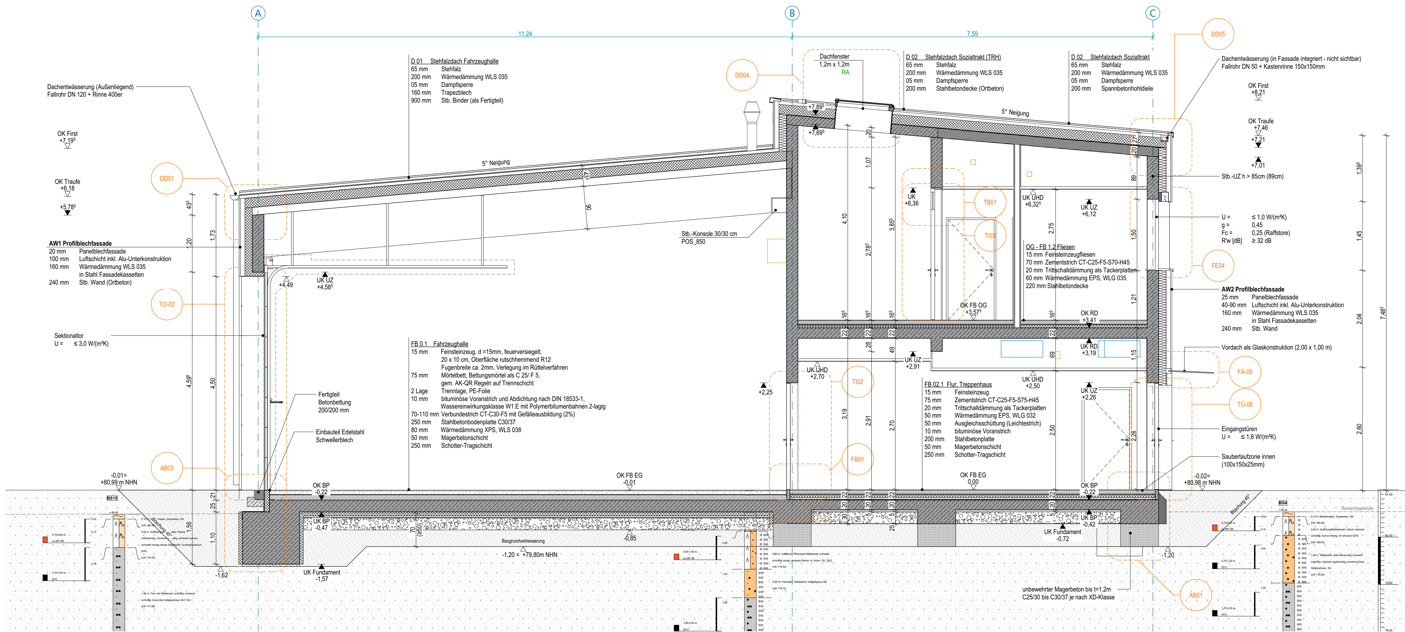
Schnitt BB
