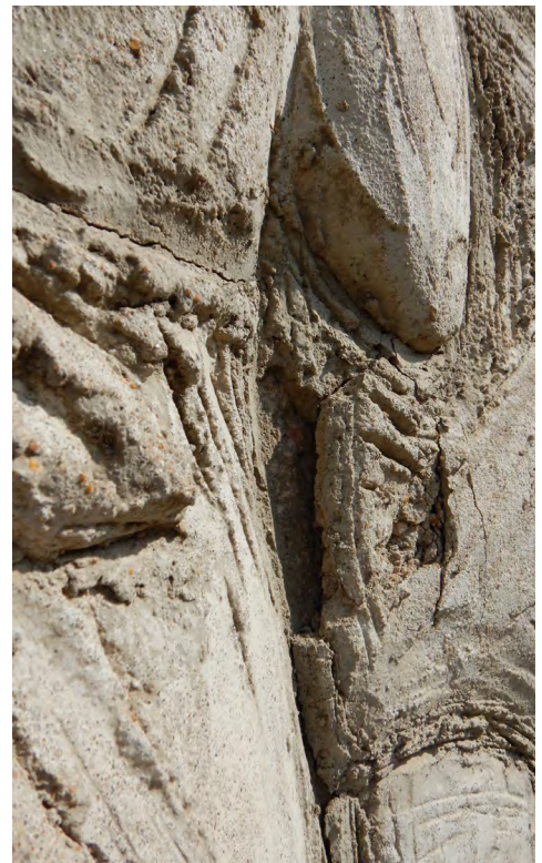
Abb. Nr.: 6 Rissbildung innerhalb der Fugen sowie eine Fehlstelle
