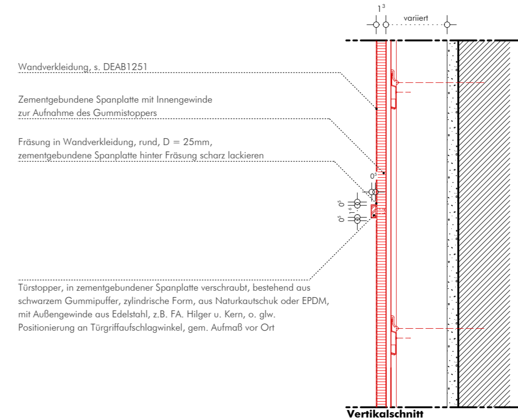
Einbau: Wandtürstopper (O1.252)
