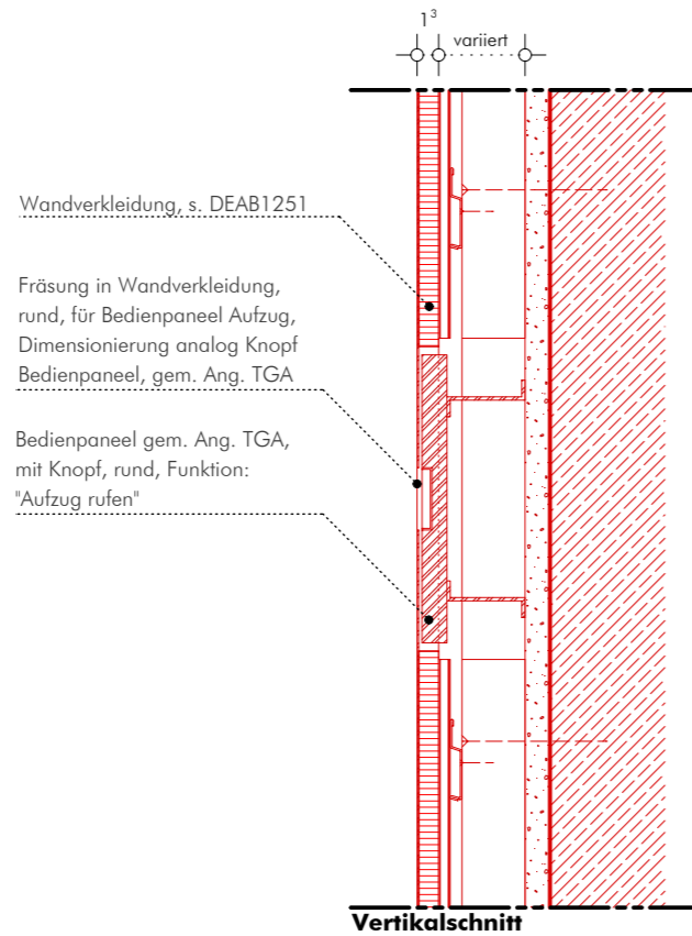
Einbau: Bedienpaneel Aufzug
