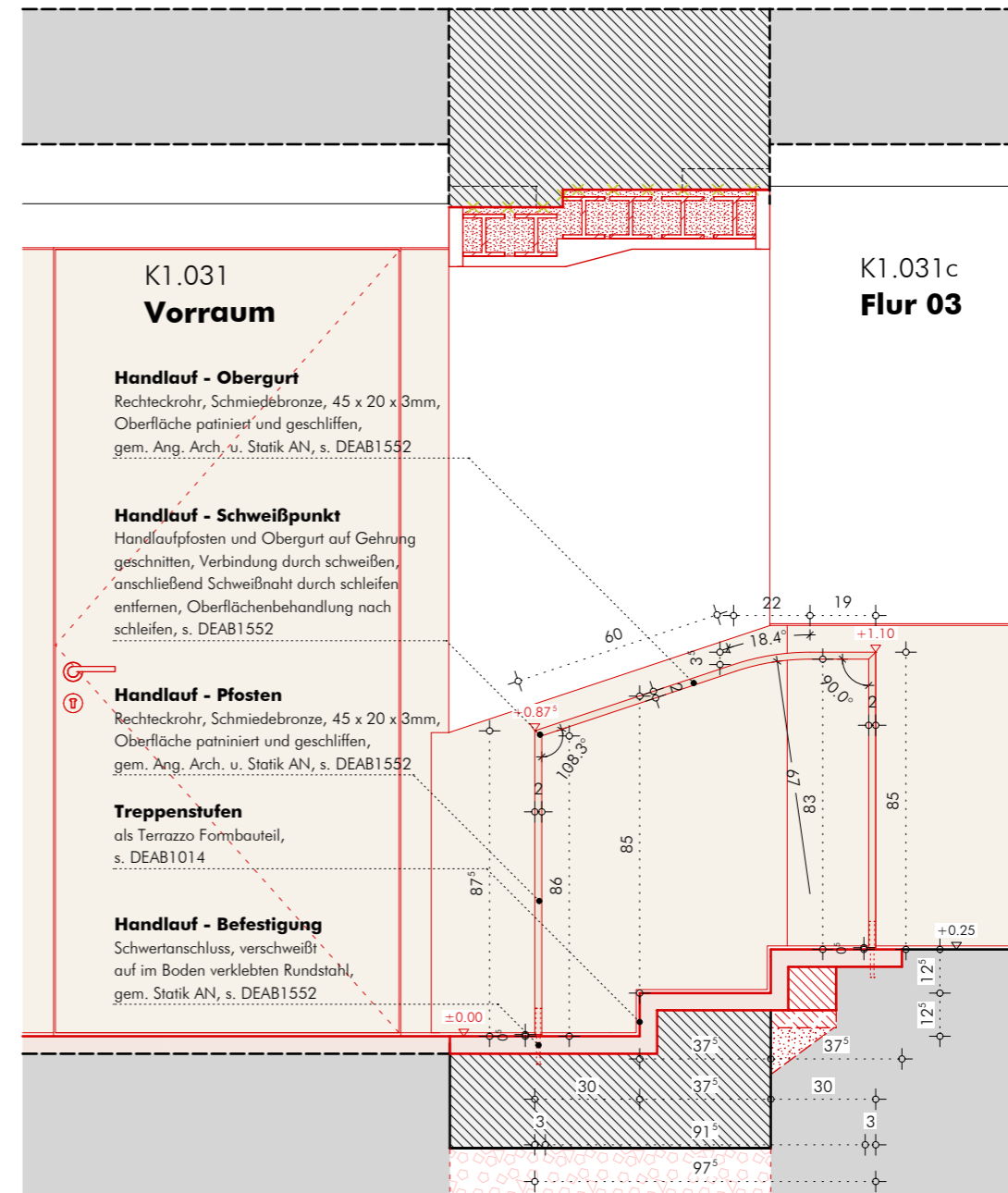
Vertikalschnitt A
