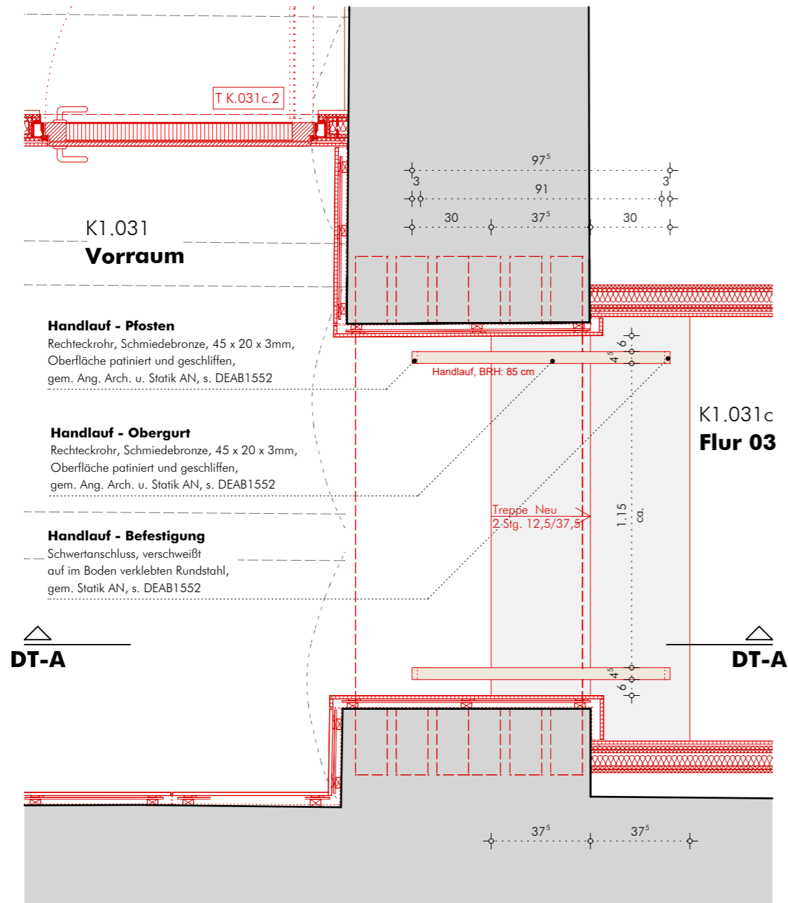
Grundriss (Ausschnitt Sockelgeschoss)
