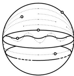
GLOBAL COMMONS
