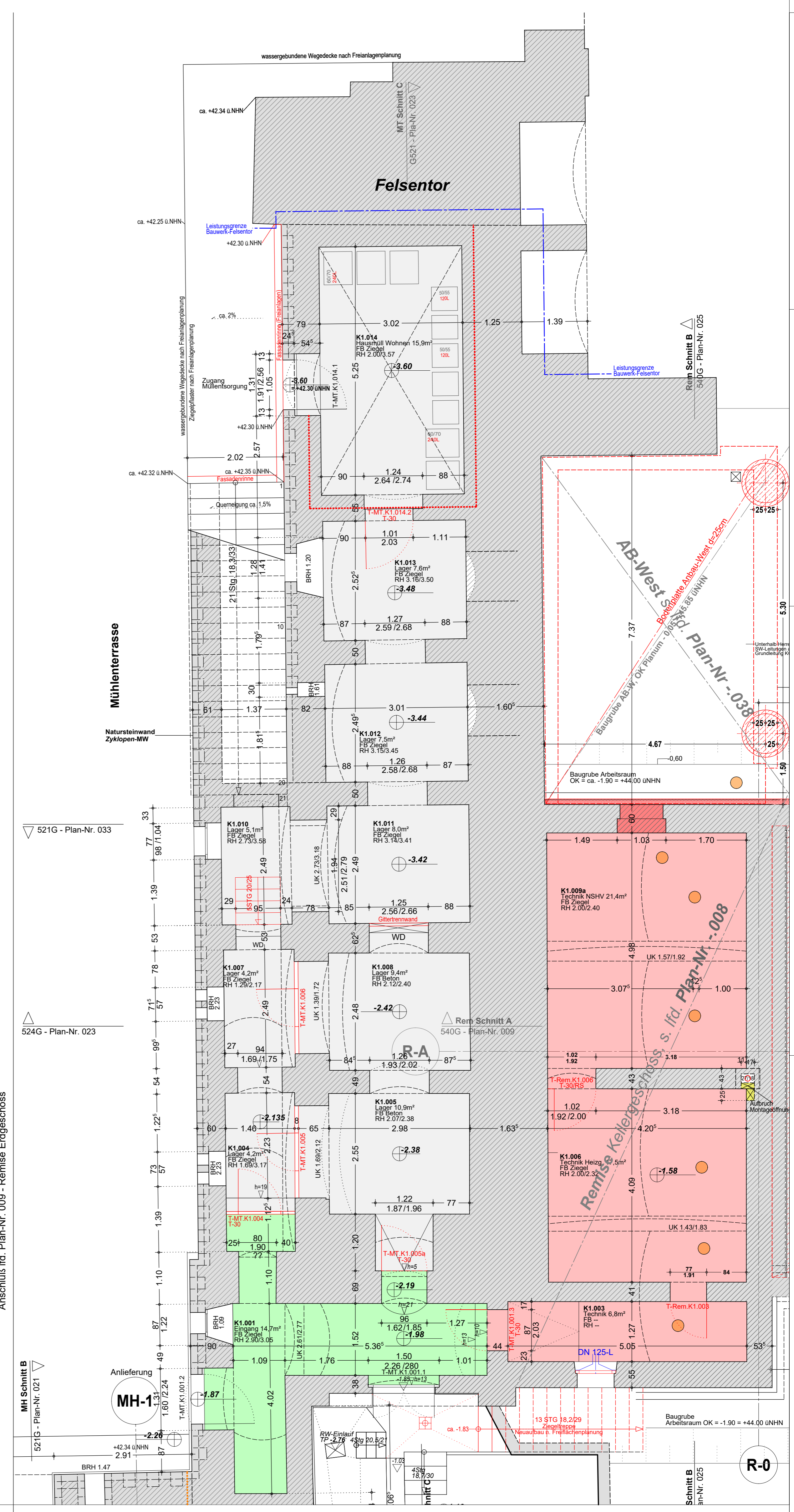
Anschluss lfd. Plan-Nr. 002 - Mühlenterrasse Erdgeschoss
