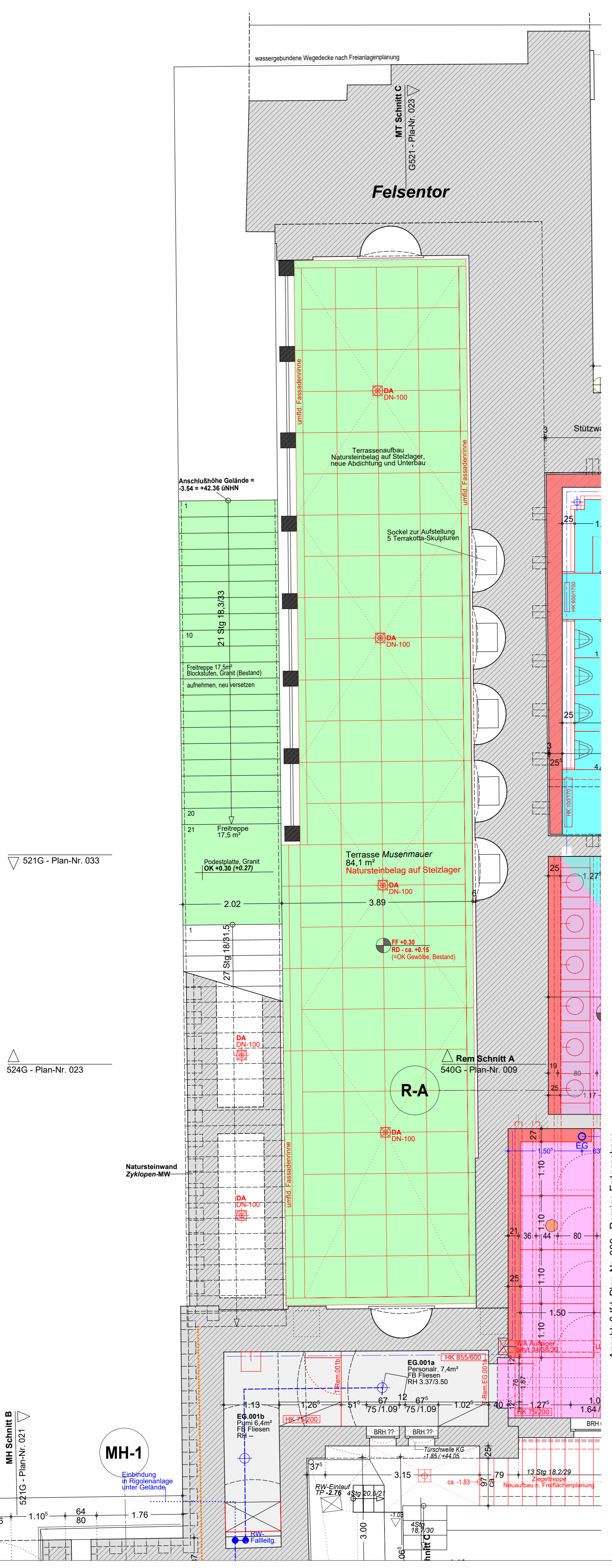
Anschluss lfd. Plan-Nr. 003 - Mühlenterrasse 1. Obergeschoss
