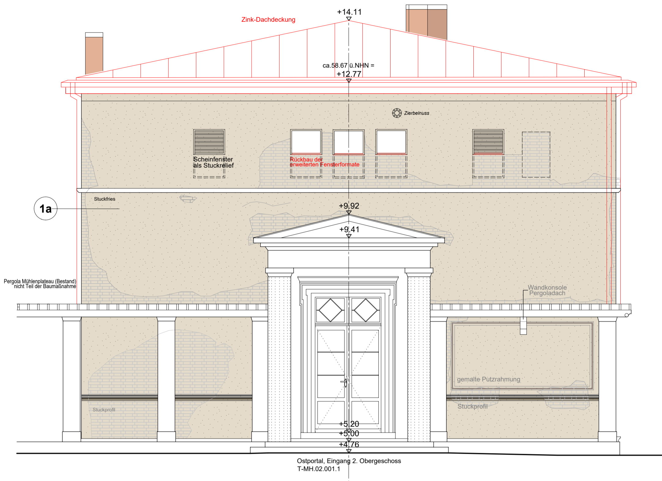
Mühlenhaus - Ansicht Ostfassade
