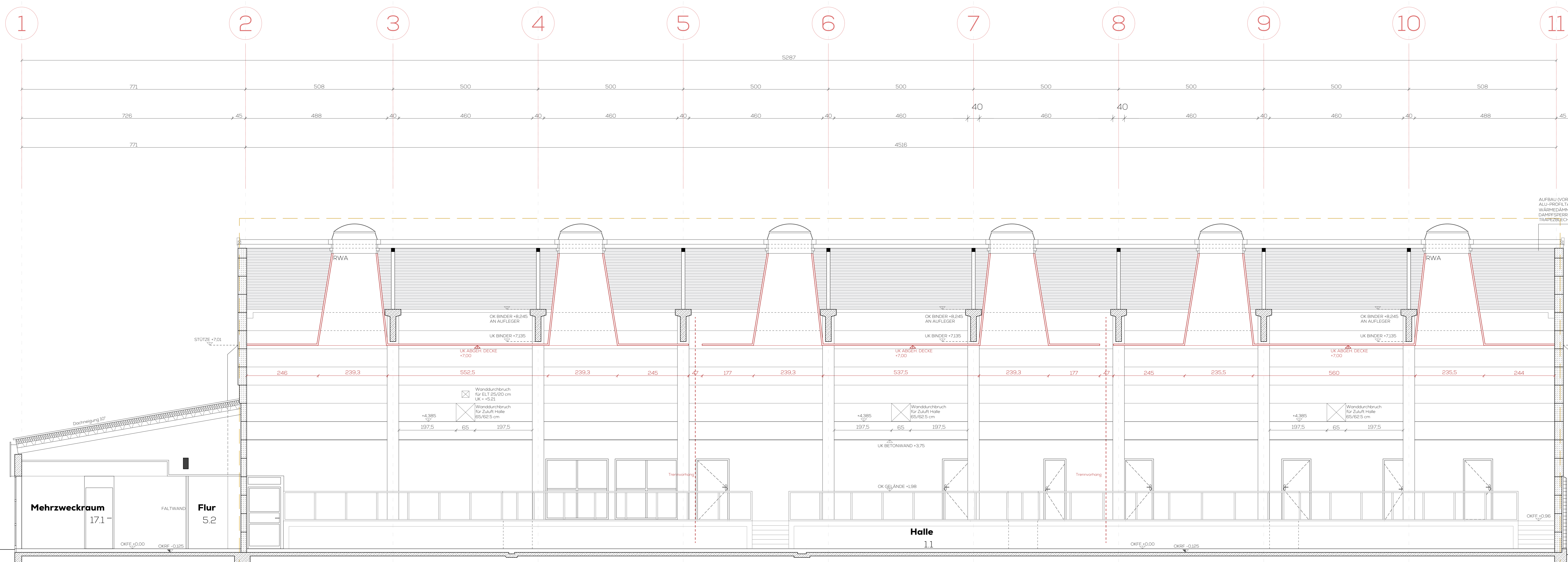
Schnitt BB
