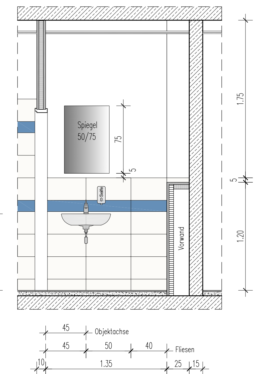
B 3.2-1 WC-Herren Ansicht 4 M 1:25
