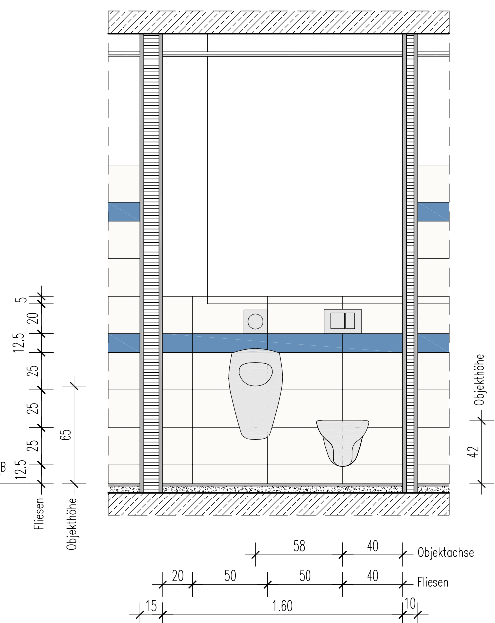
B 3.2-1 WC-Herren Ansicht 5 M 1:25
