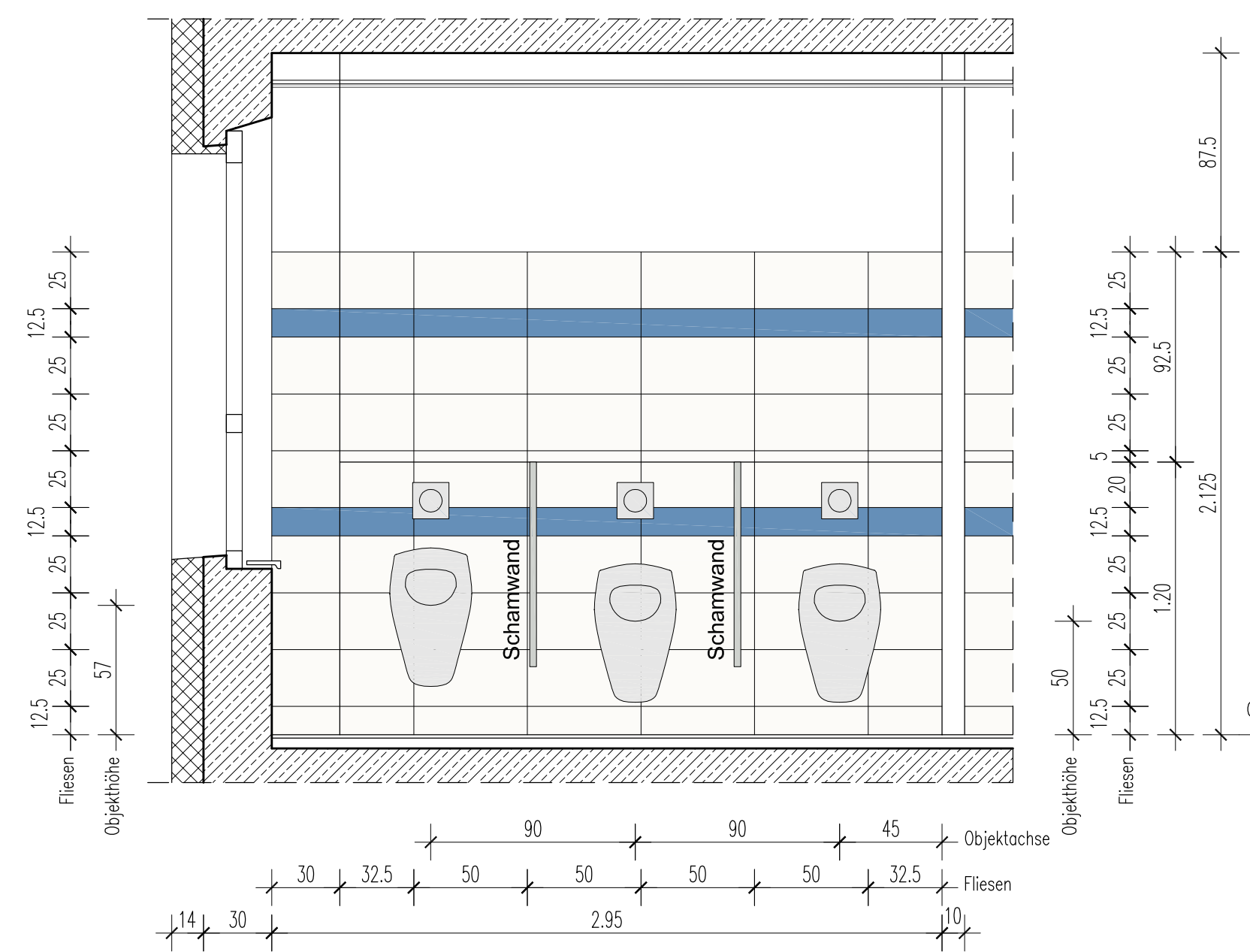
B 3.2 WC-Jungen Ansicht 7 M 1:25
