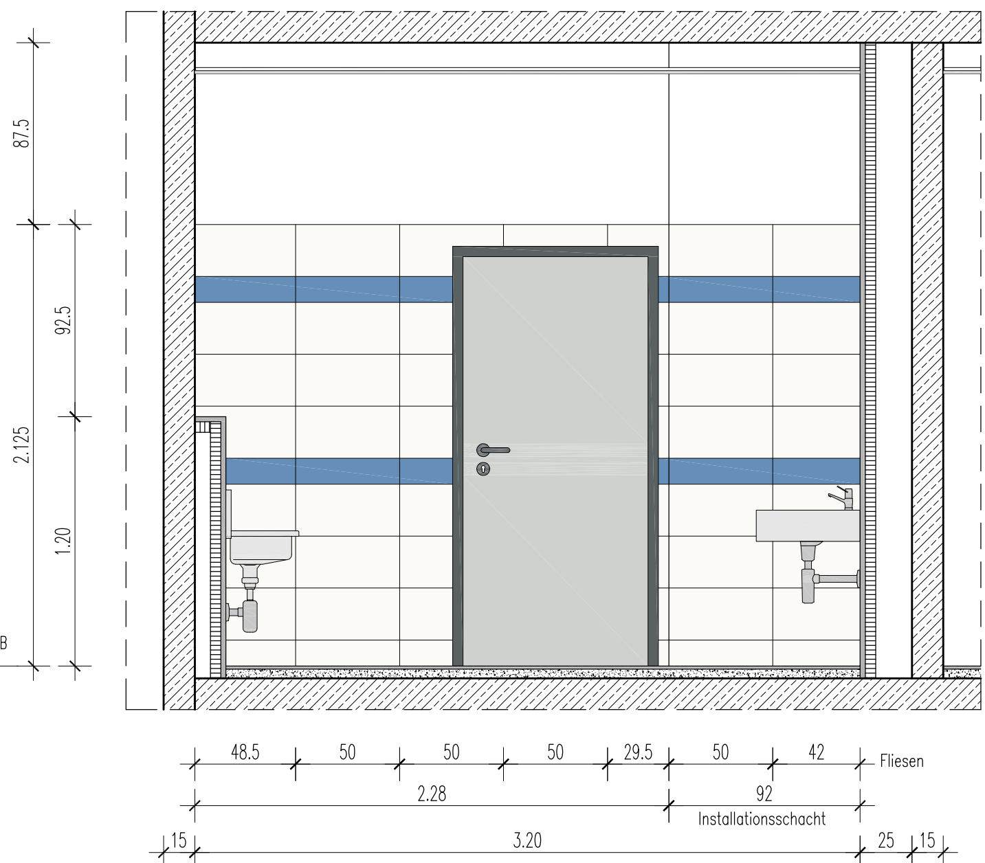
B 3.3 Vorraum Ansicht 2 M 1:25
