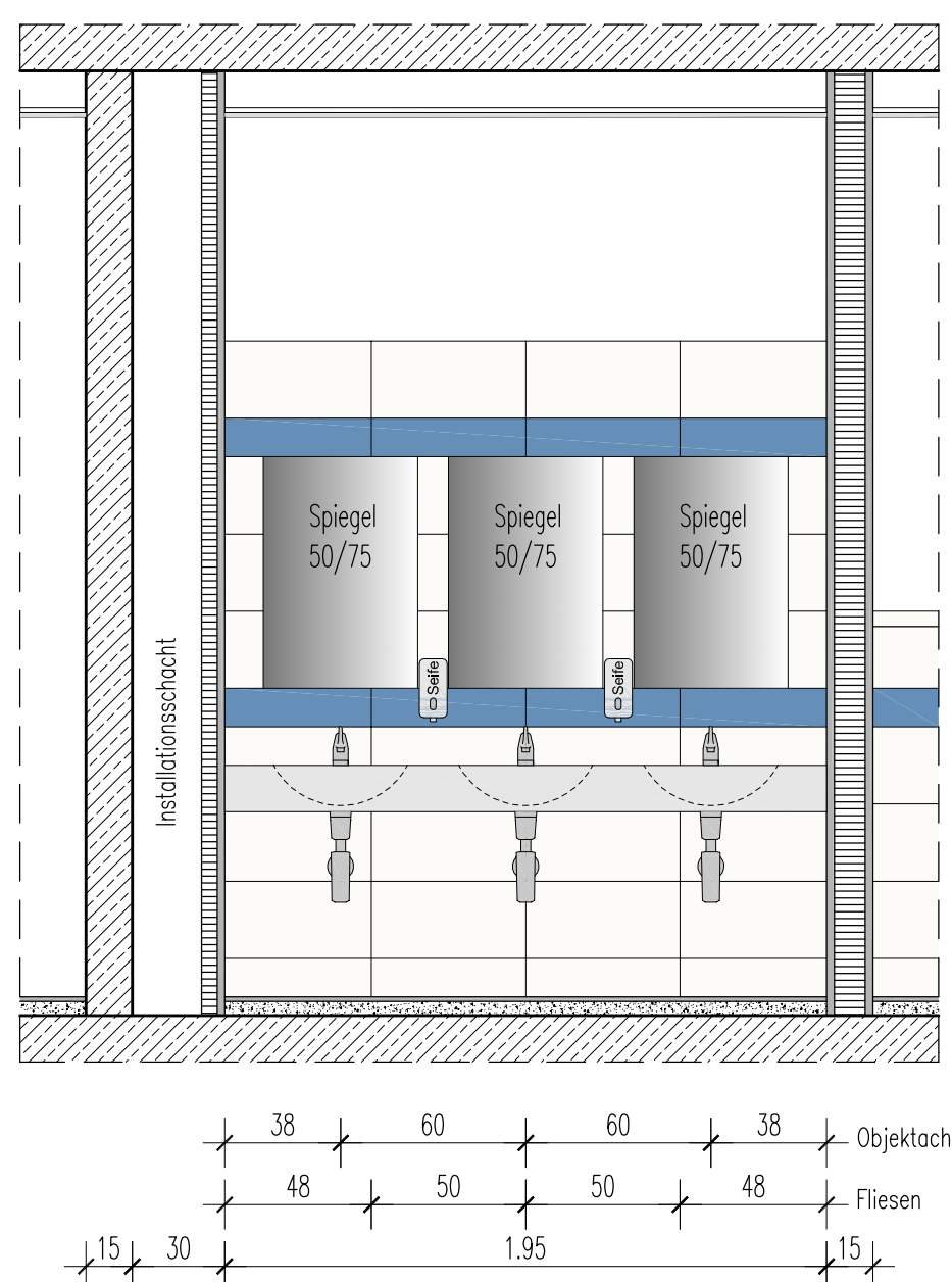
B 3.3 Vorraum Ansicht 3 M 1:25
