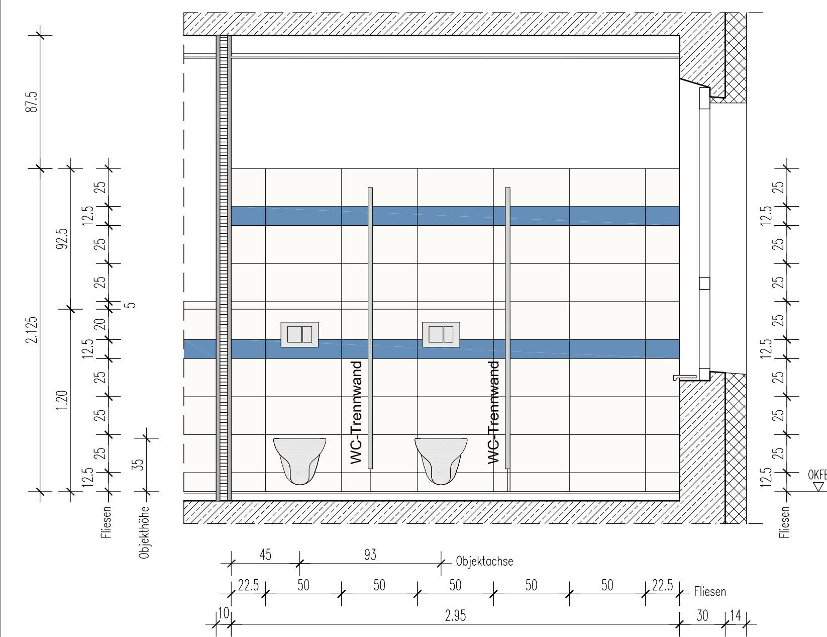
B 3.2 WC-Jungen Ansicht 6 M 1:25
