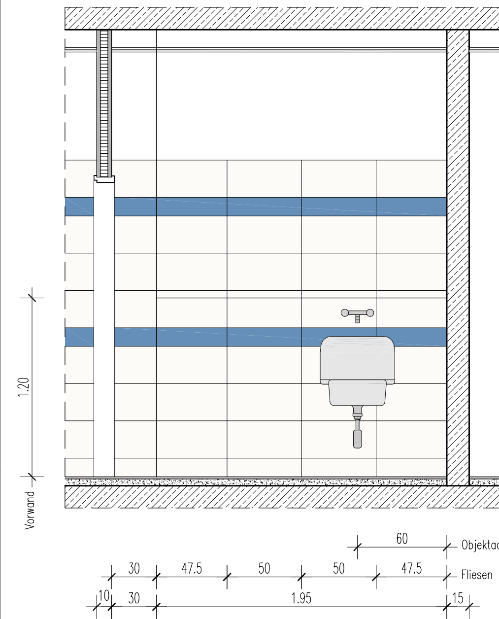
B 3.3 Vorraum Ansicht 1 M 1:25
