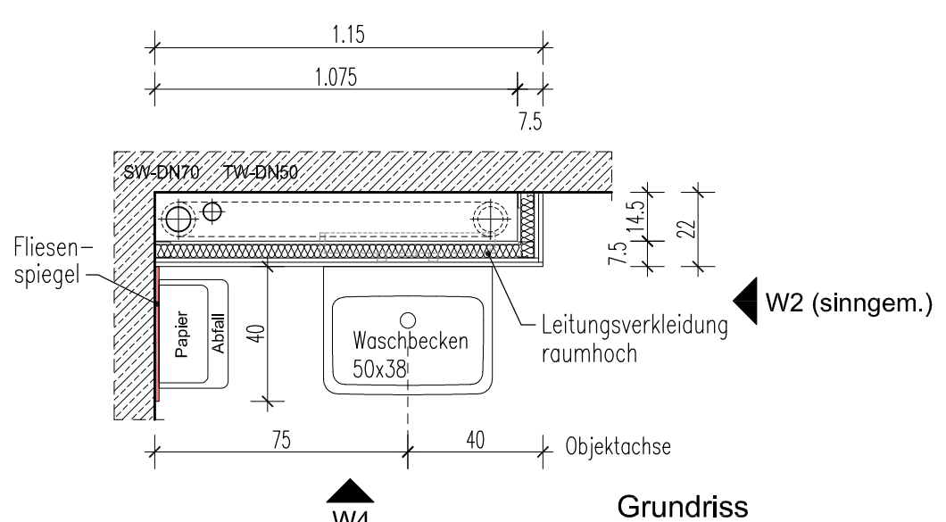
Grundriss
