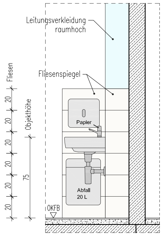
Ansicht W2
