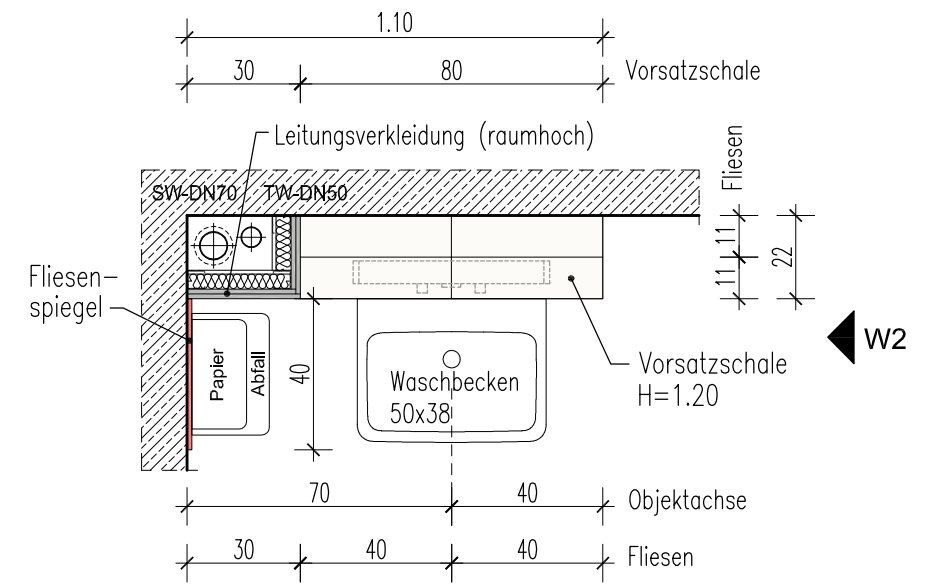
Grundriss
