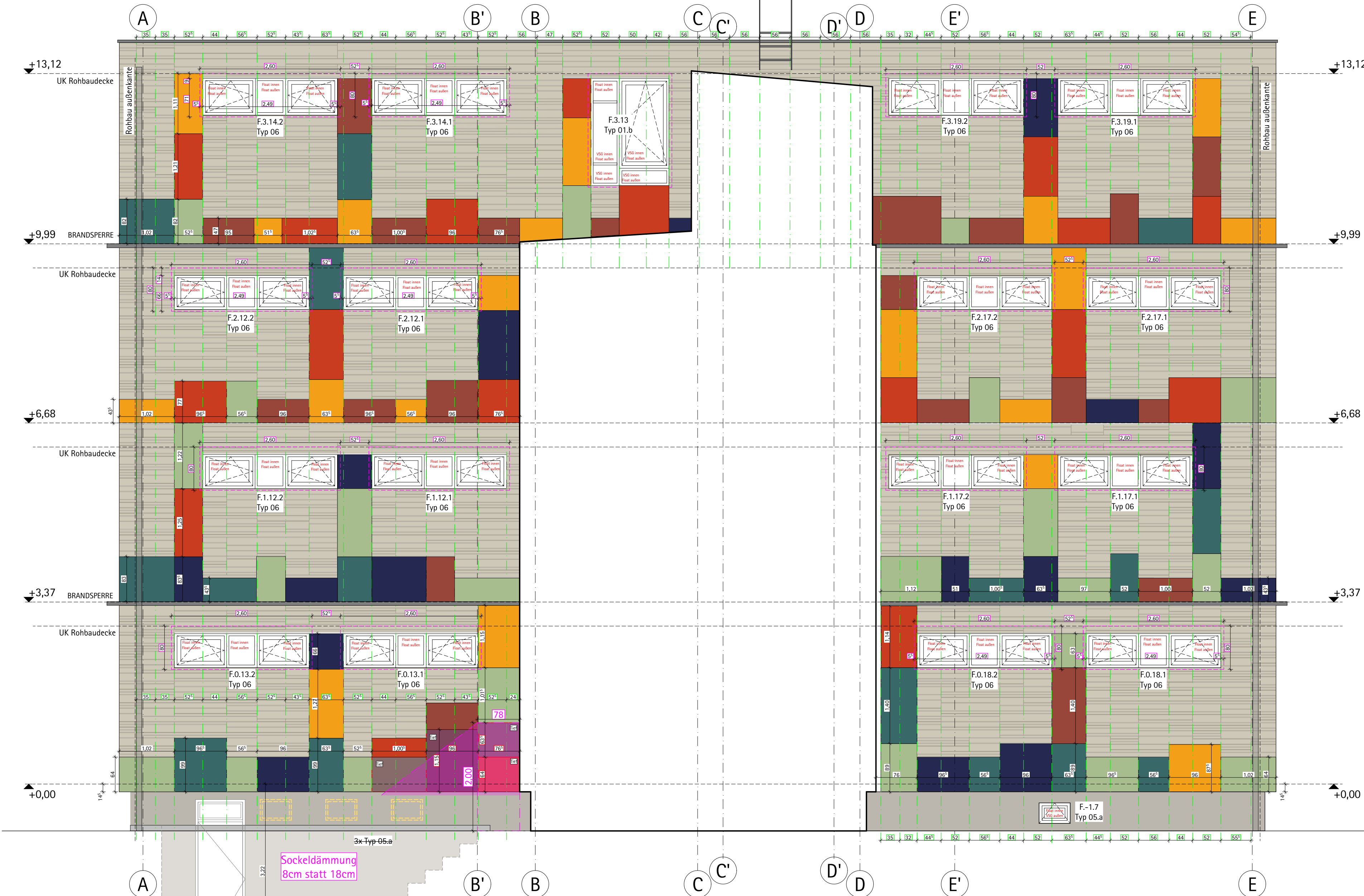
ANSICHT NORD (H-Bau Fassade innen)
