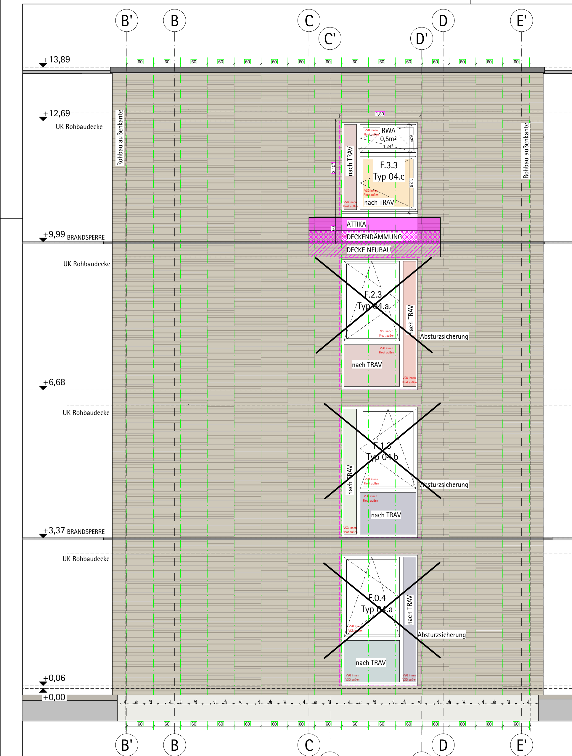
ANSICHT NORD (Treppenhaus)
