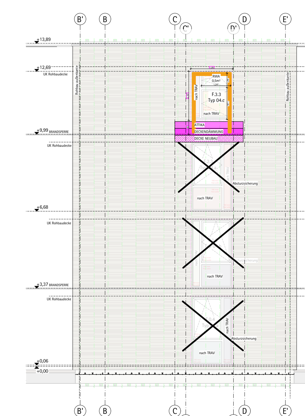
LEIBUNGSFARBE Ansicht Nord (Treppenhaus)
