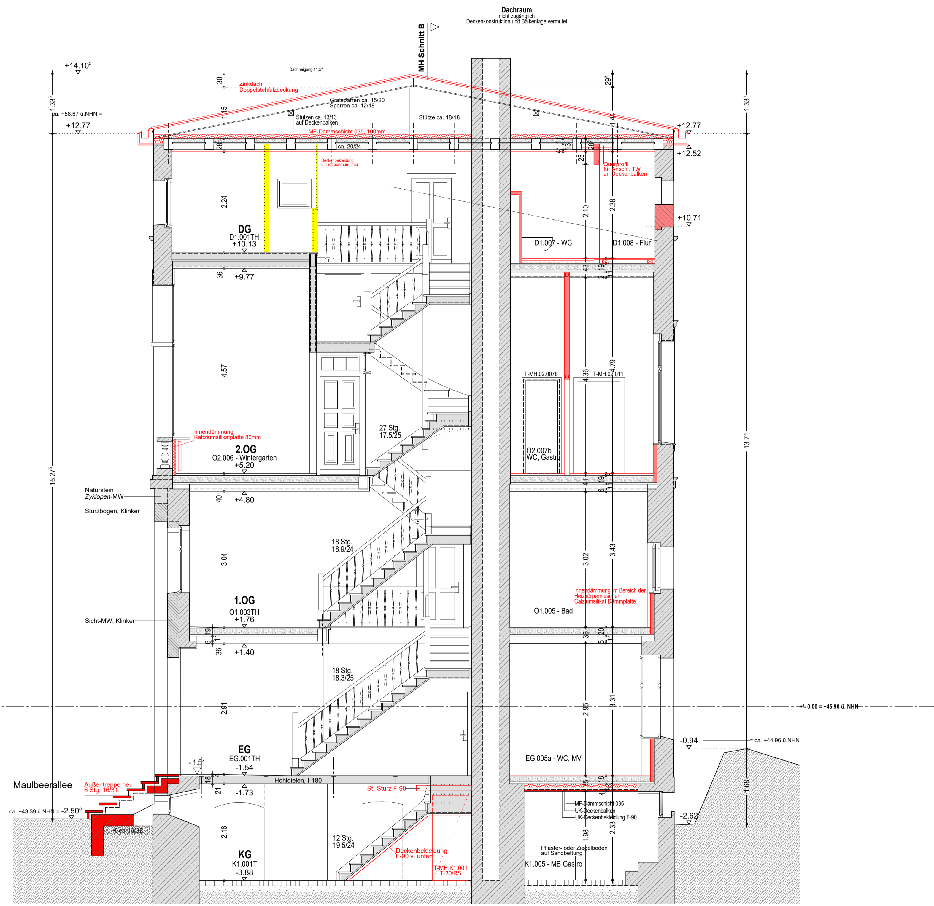
MH Schnitt B 52/IG - Plan-Nr. 021 MH-1
