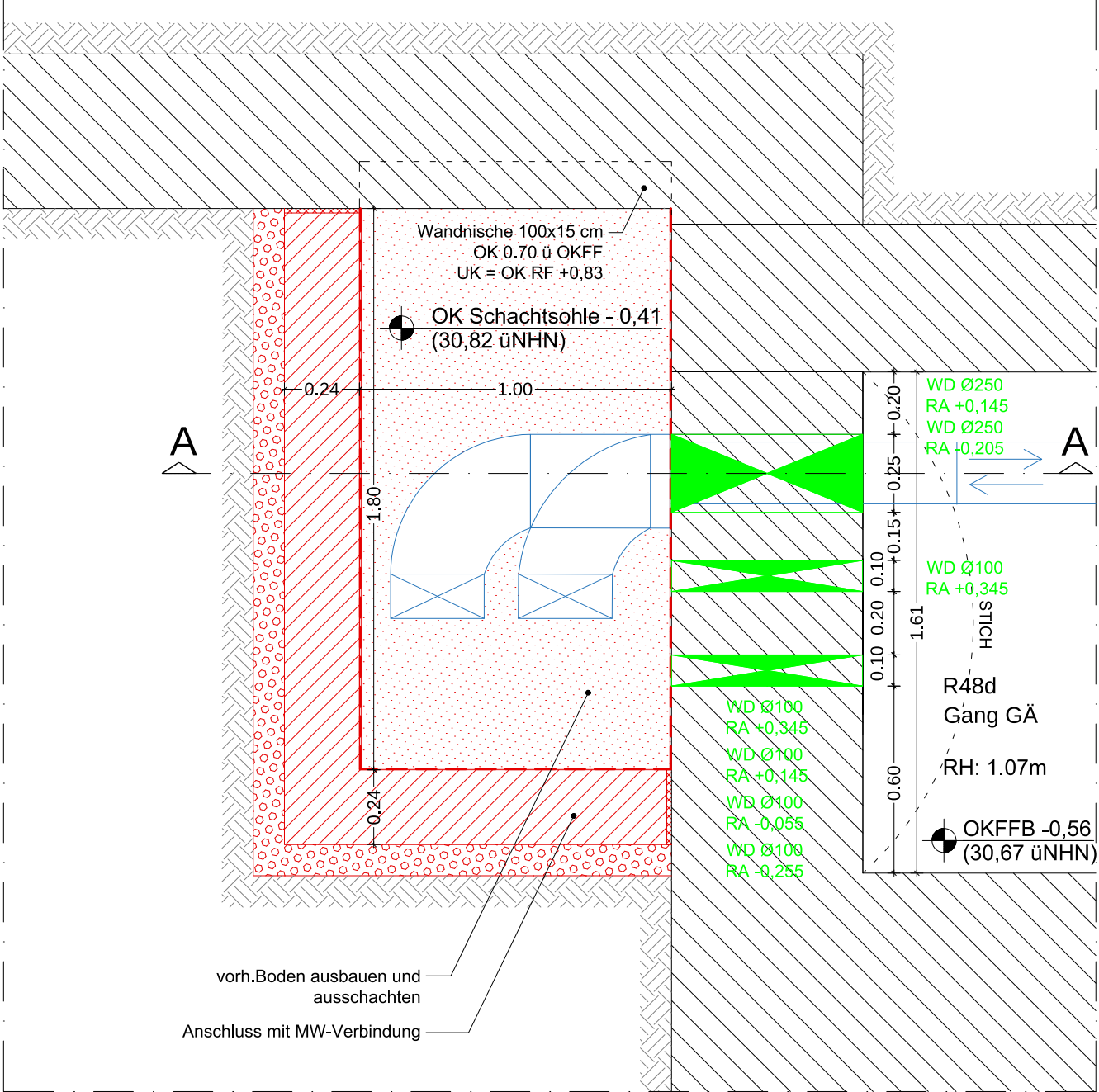
Grundriss KG M 1:20
