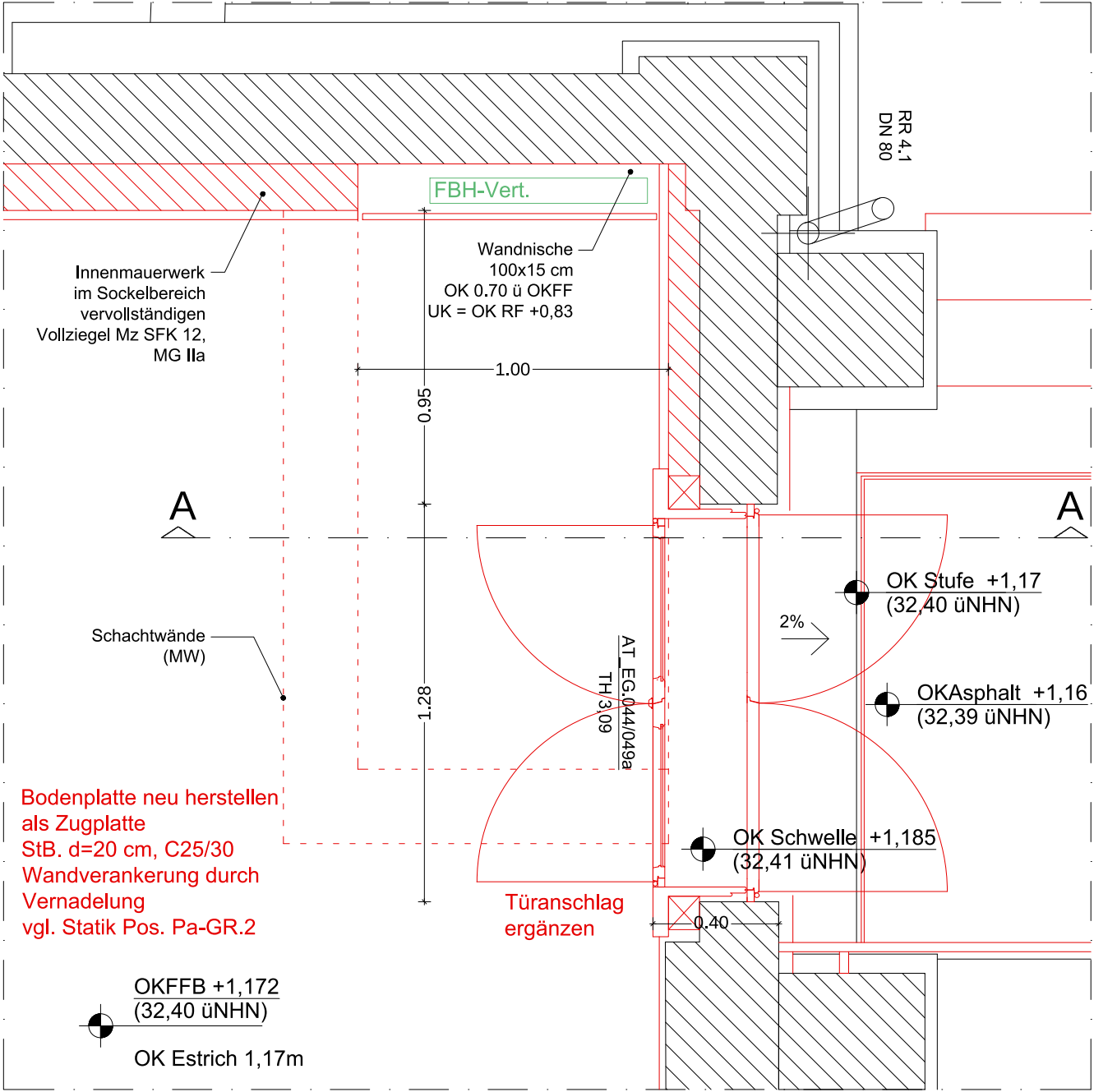
Grundriss EG M 1:20
