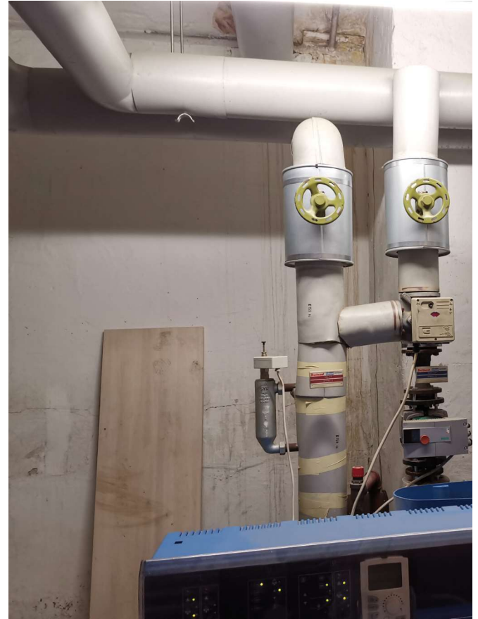
gedämmte Verteiler im UG Heizraum
