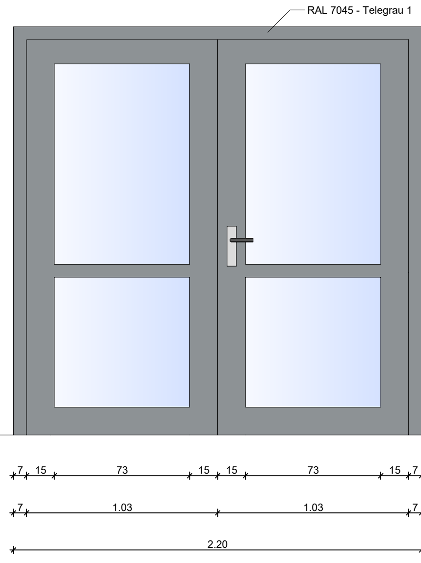
Eingangstüren - Ansicht innen
