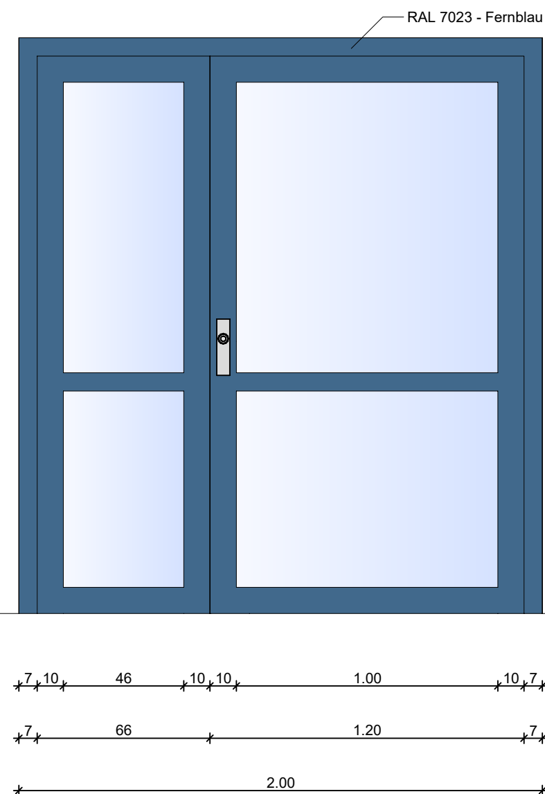
Türen Giebelwände (Fluchttreppen) - Ansicht außen
