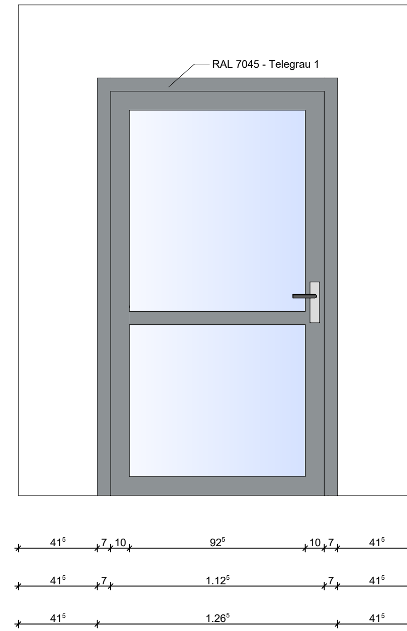
Türen in Brandwänden
