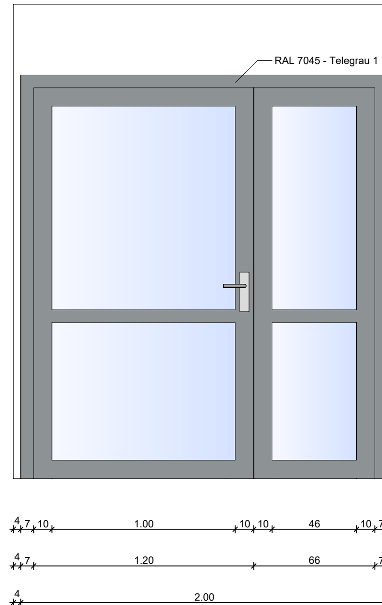
Türen Giebelwände (Fluchttreppen) - Ansicht innen
