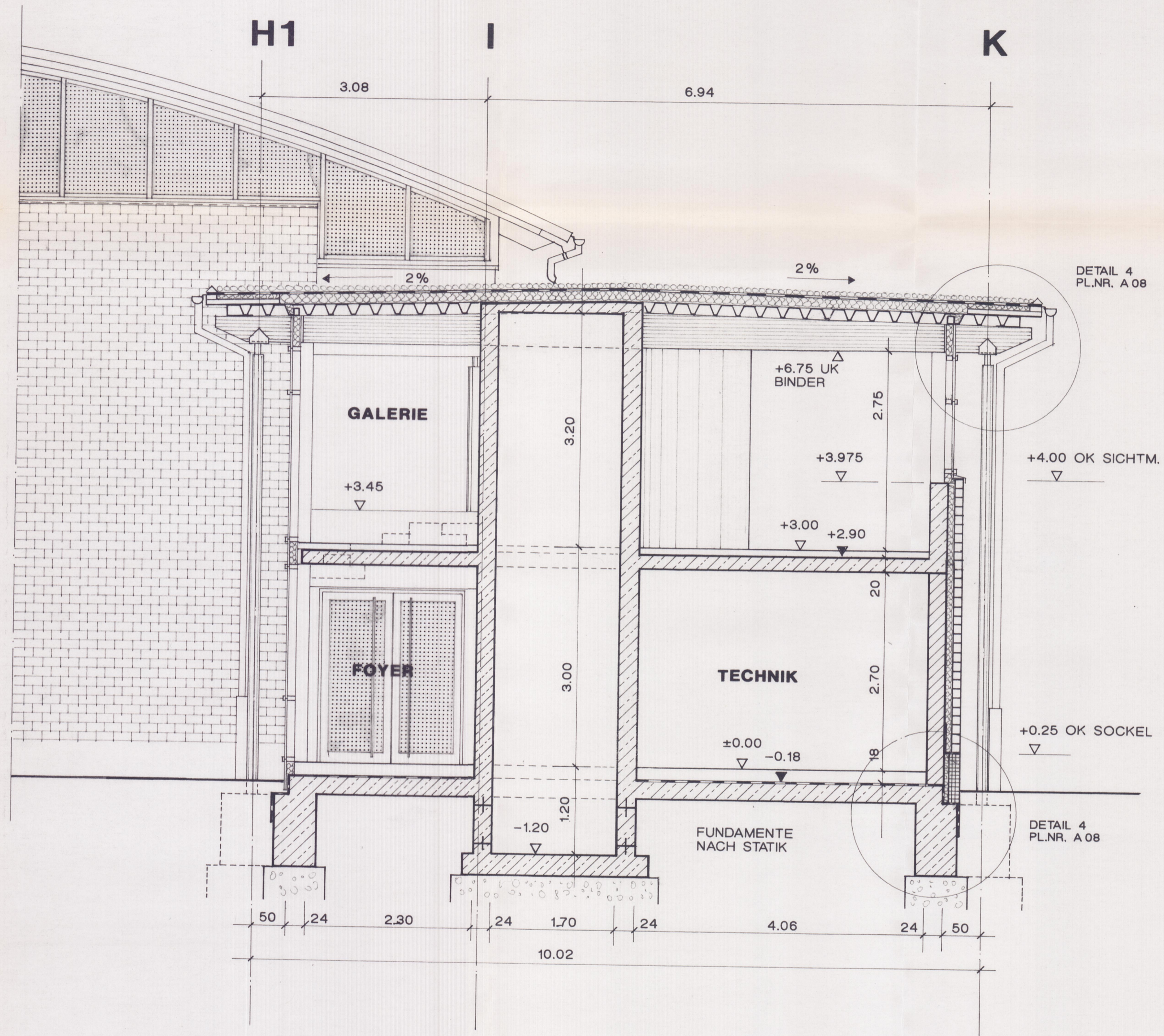
SCHNITT B-B
