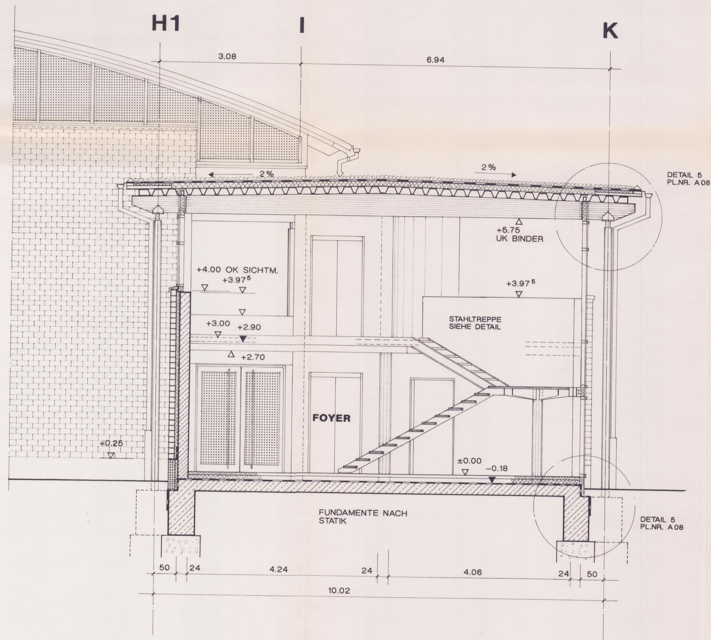
SCHNITT C-C
