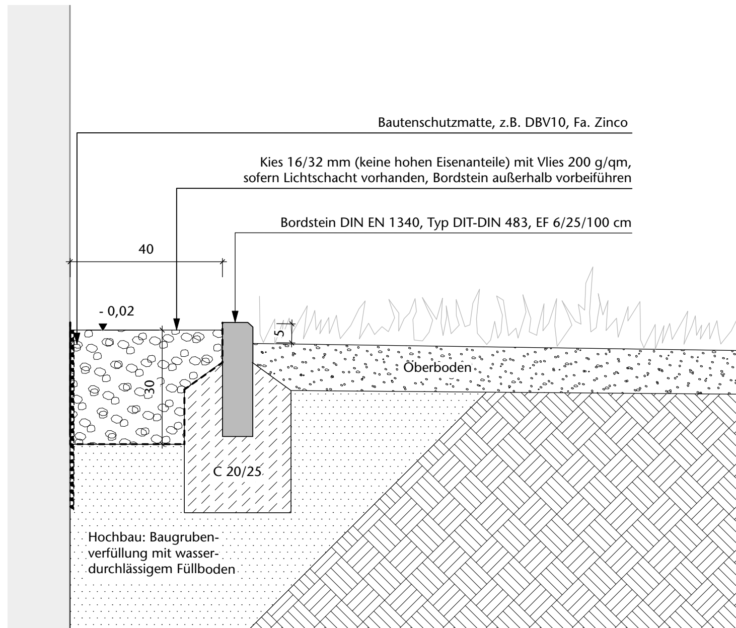
Traufkiesstreifen M. 1:10
