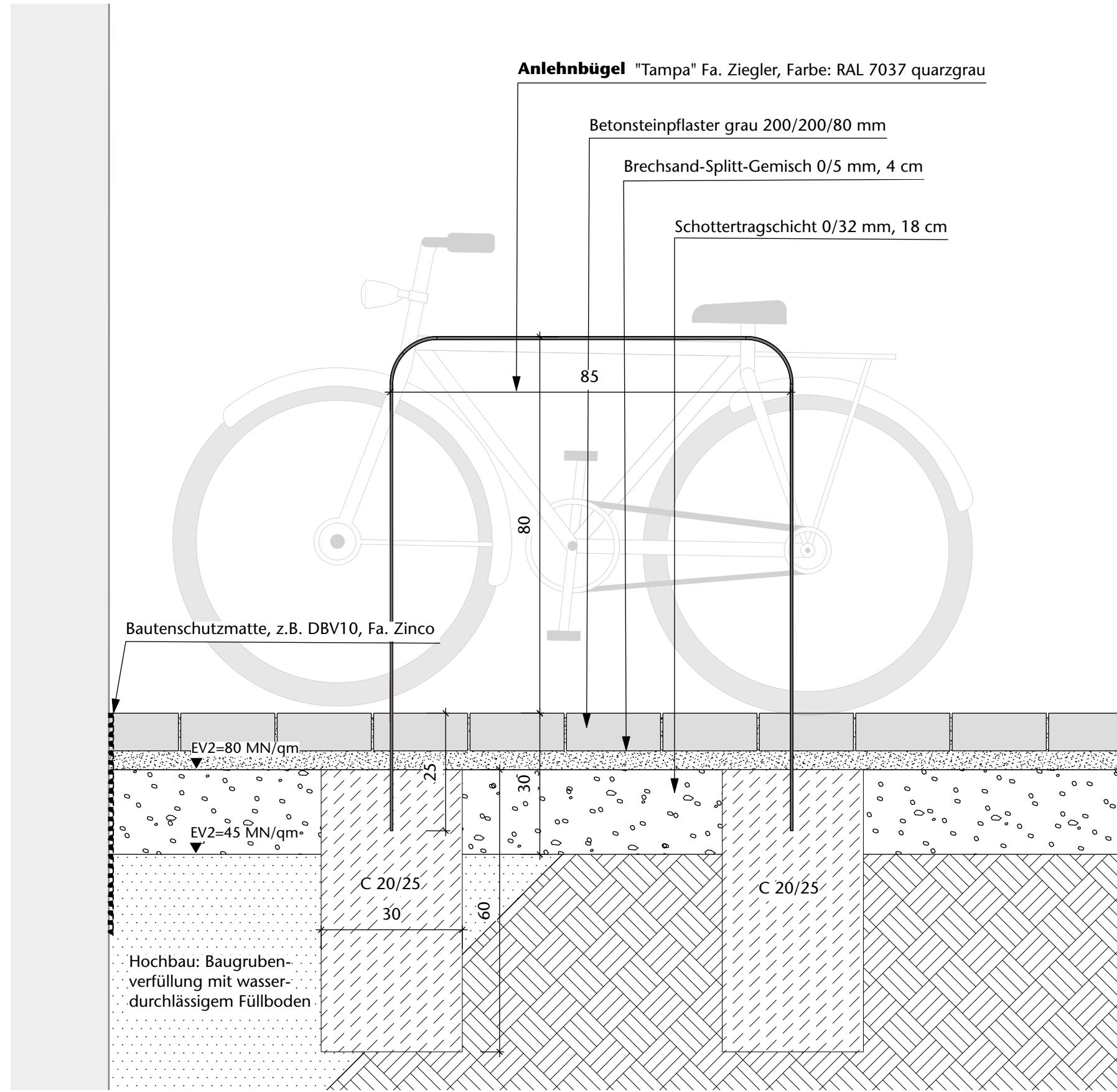
Fahrradstellplatz M. 1 : 10
