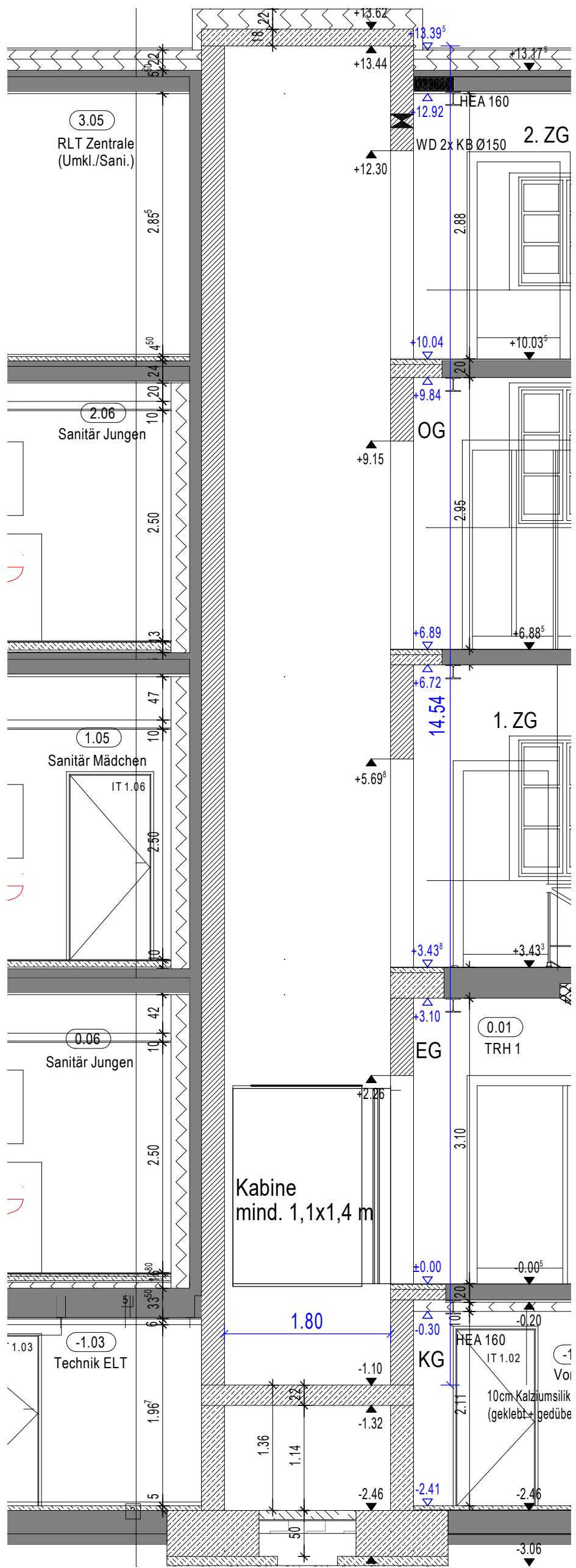
Schachtlängsschnitt
