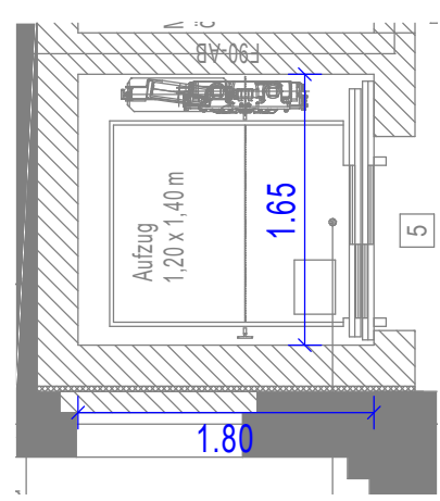
Schachtquerschnitt
