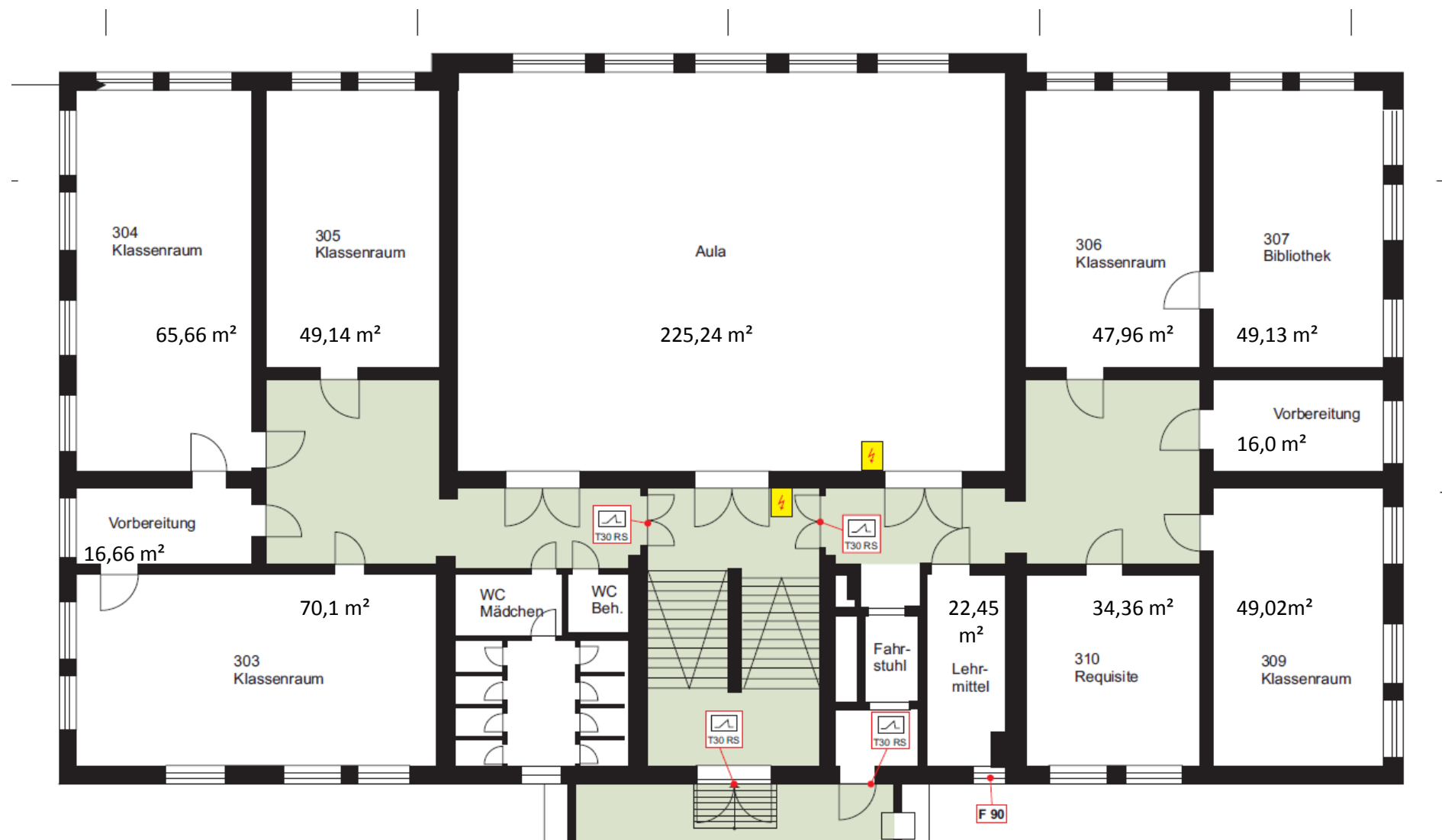
Gymnasium Altbau 2. OG
