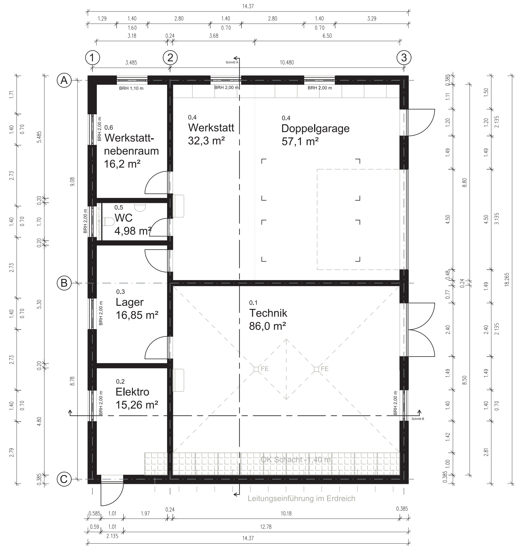
Grundriss
