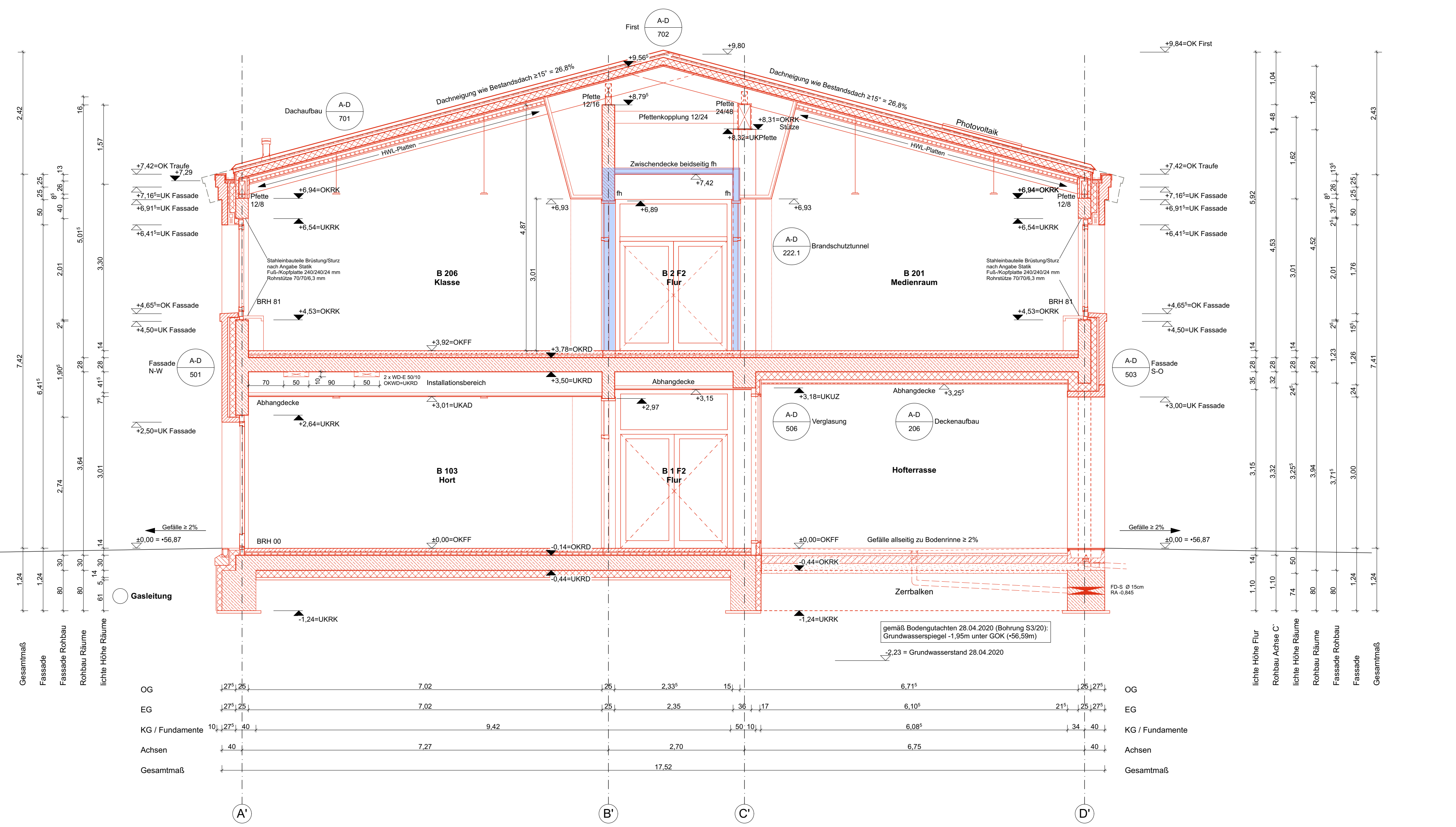
Schnitt 02
