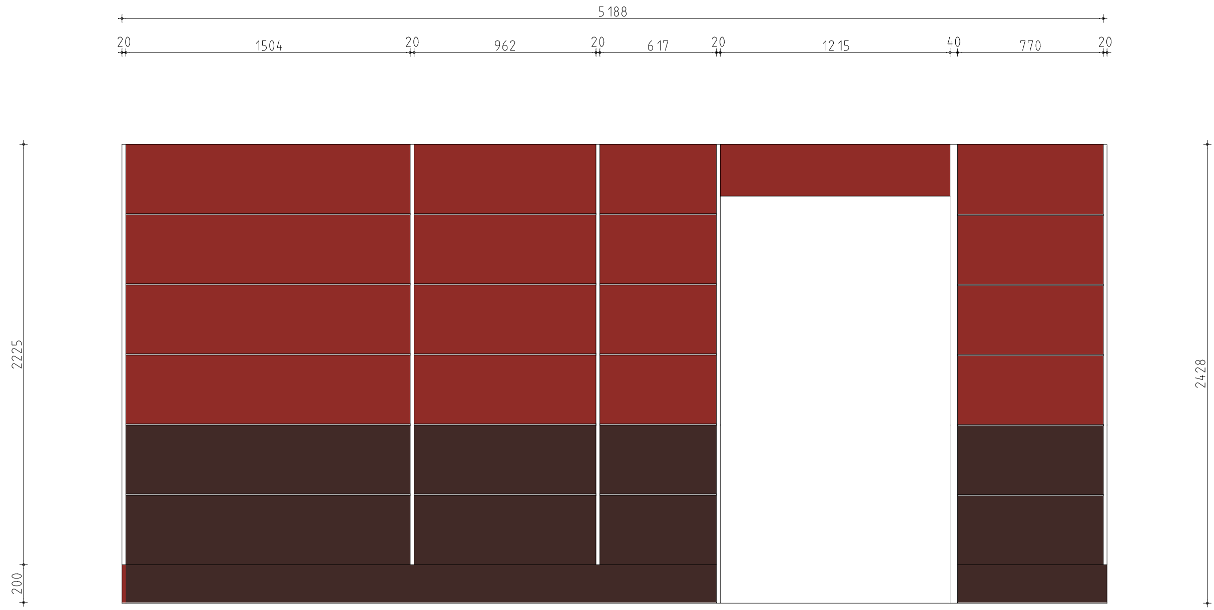
Ansicht Rückwand Bistrotresen
