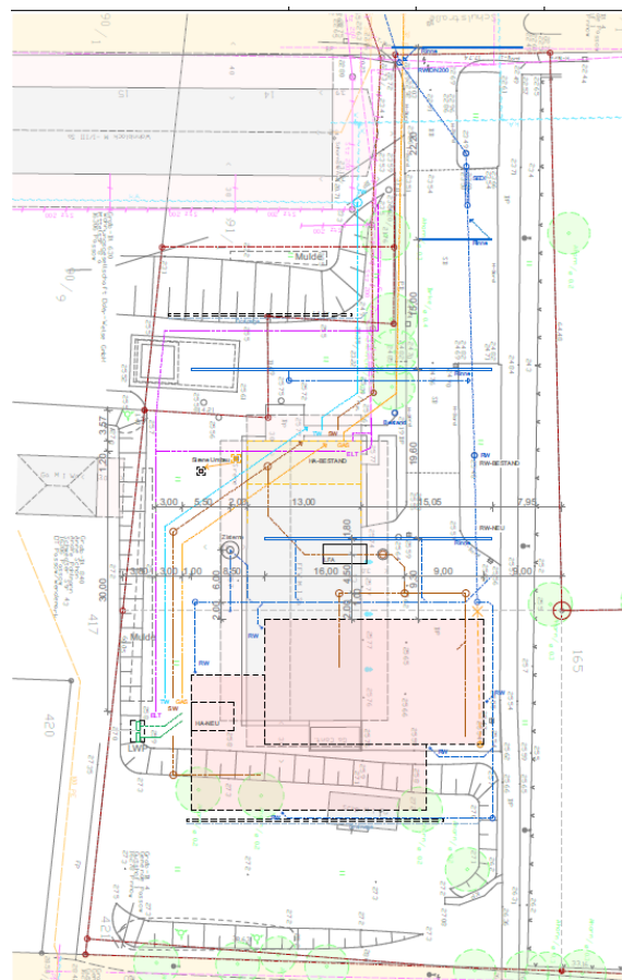
Planung Neubau Feuerwehrgebäude Passow (Bestand verblasst hinterlegt)
